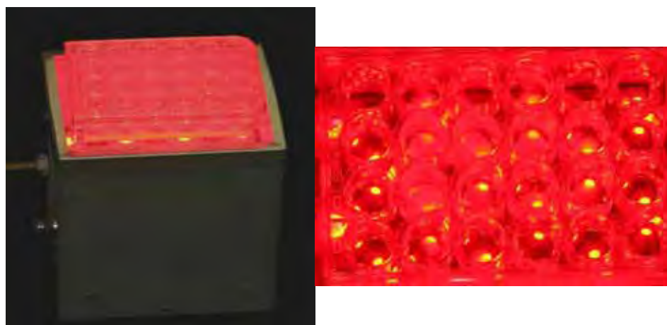
FIGURA 6 – Placa de 24 compartimentos posicionada sobre a superfície de iluminação da “Bio Table” vermelha acionada.
