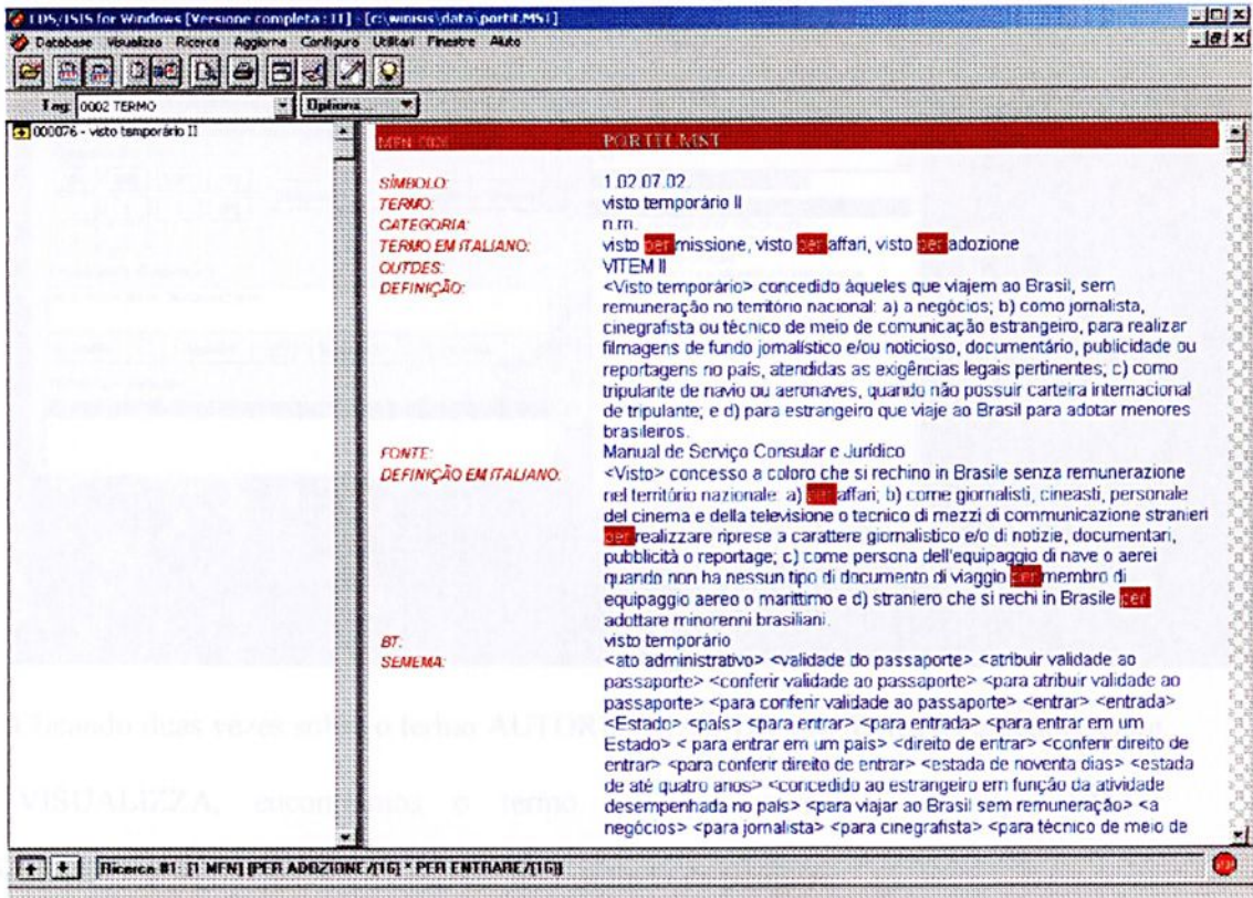
Figura 18. CDS/ISIS: Resultado da busca onomasiológica (português-italiano)
