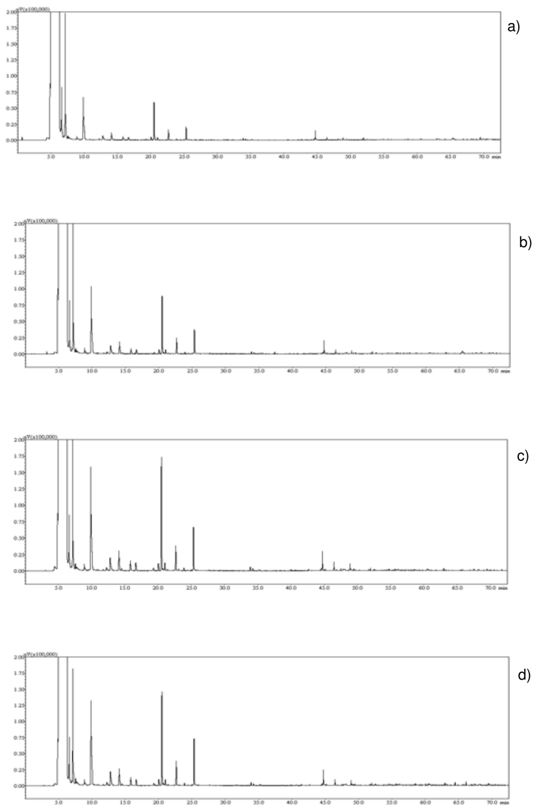
Figura 12. Cromatograma dos compostos voláteis da uvaia capturados por 1 hora (a), 2 horas (b), 3 horas (c) e 4 horas (d), eluídos com hexano e separados na coluna DB-5.
