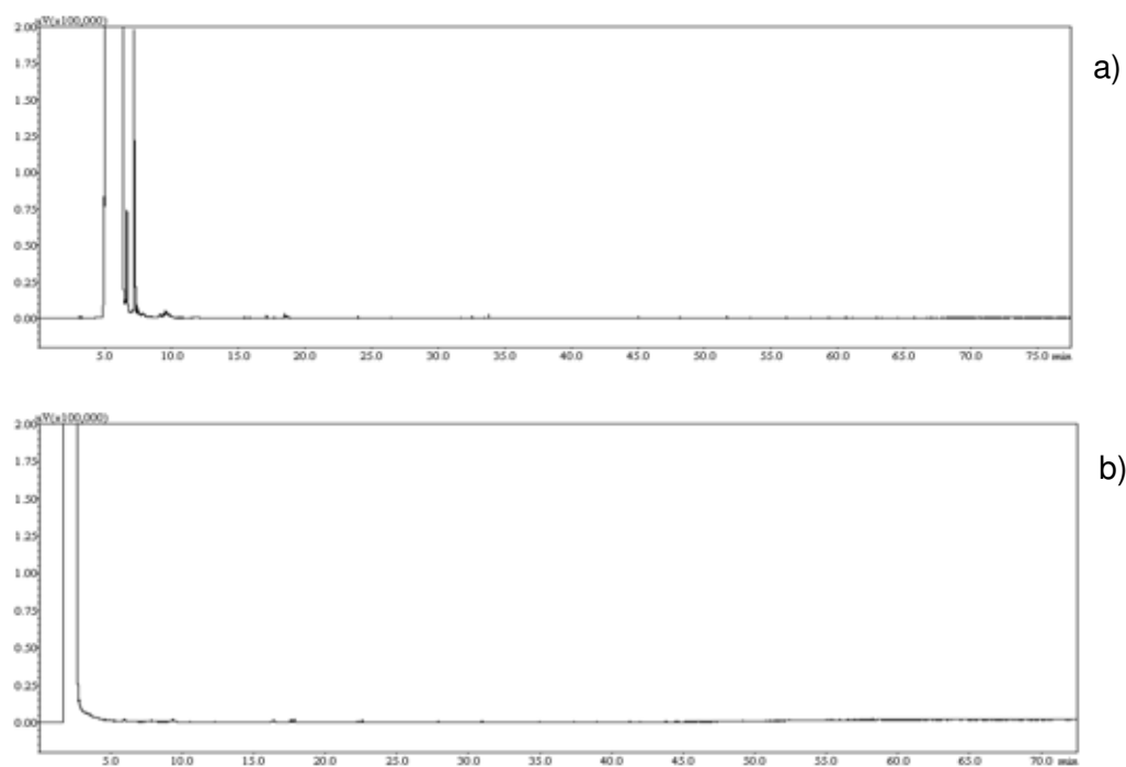
Figura 7. Cromatograma do solvente hexano nas colunas DB-5 (a) e DB-Wax (b).
