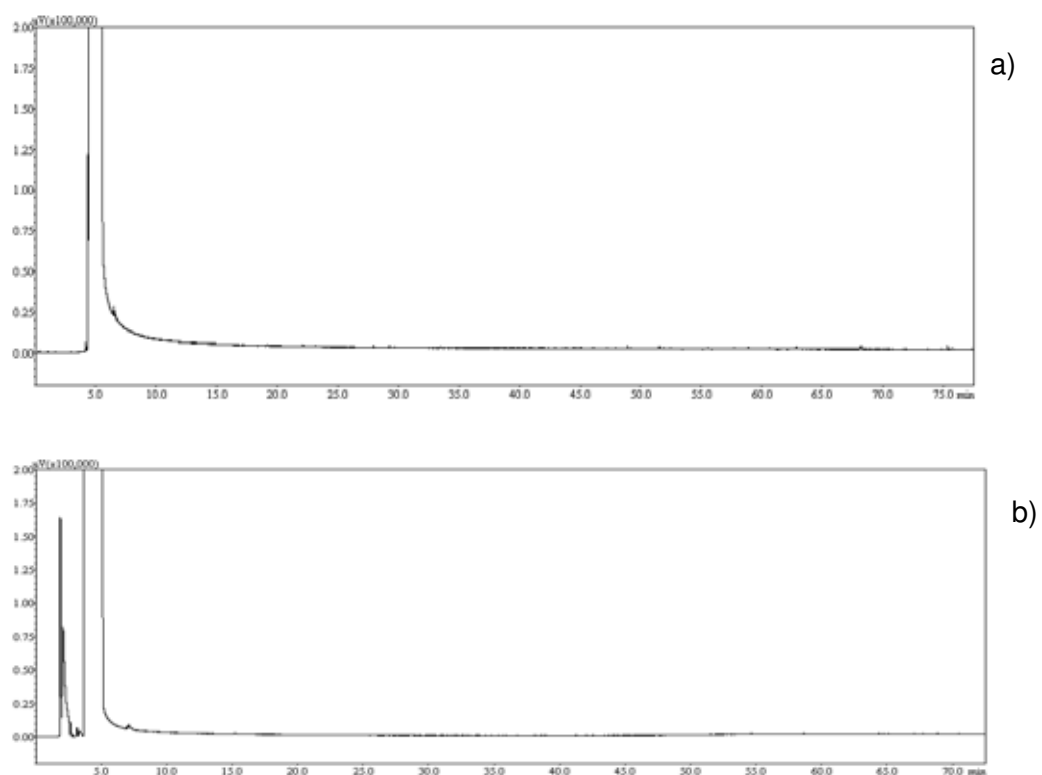
Figura 8. Cromatograma do solvente diclorometano nas colunas DB-5 (a) e DB-Wax (b).
