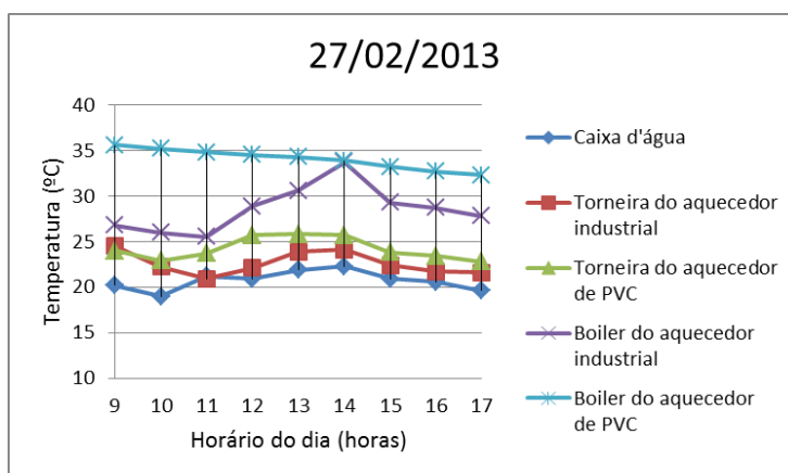
FIGURA 6 – Aquecedor solar de PVC e aquecedor solar industrial 27/02/2013.
