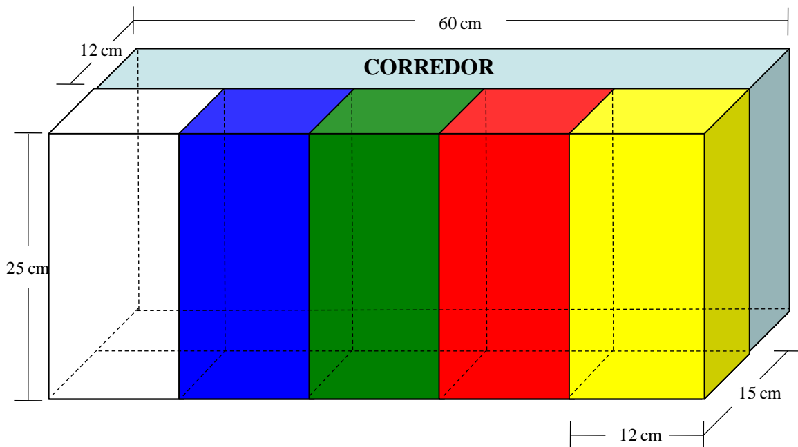
Figura 5: Esquema do aquário utilizado para avaliar a preferência por coloração ambiental.
