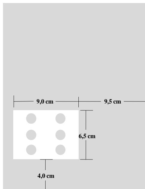
Figura 18: Posicionamento da porta (branca) na divisória (cinza) do aquário utilizado para avaliar o esforço. Círculos em cinza indicam aberturas de 1,0 cm de diâmetro.
