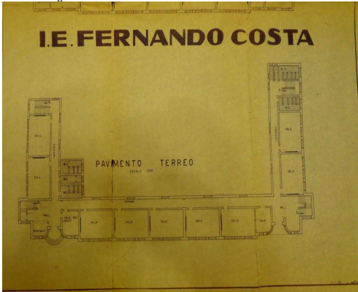
Figura 7- Planta do Pavimento térreo do IE “Fernando Costa”
