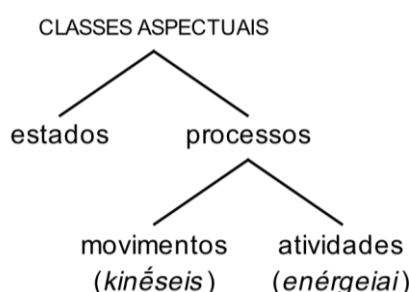
Figura 1. Classes aspectuais aristotélicas
