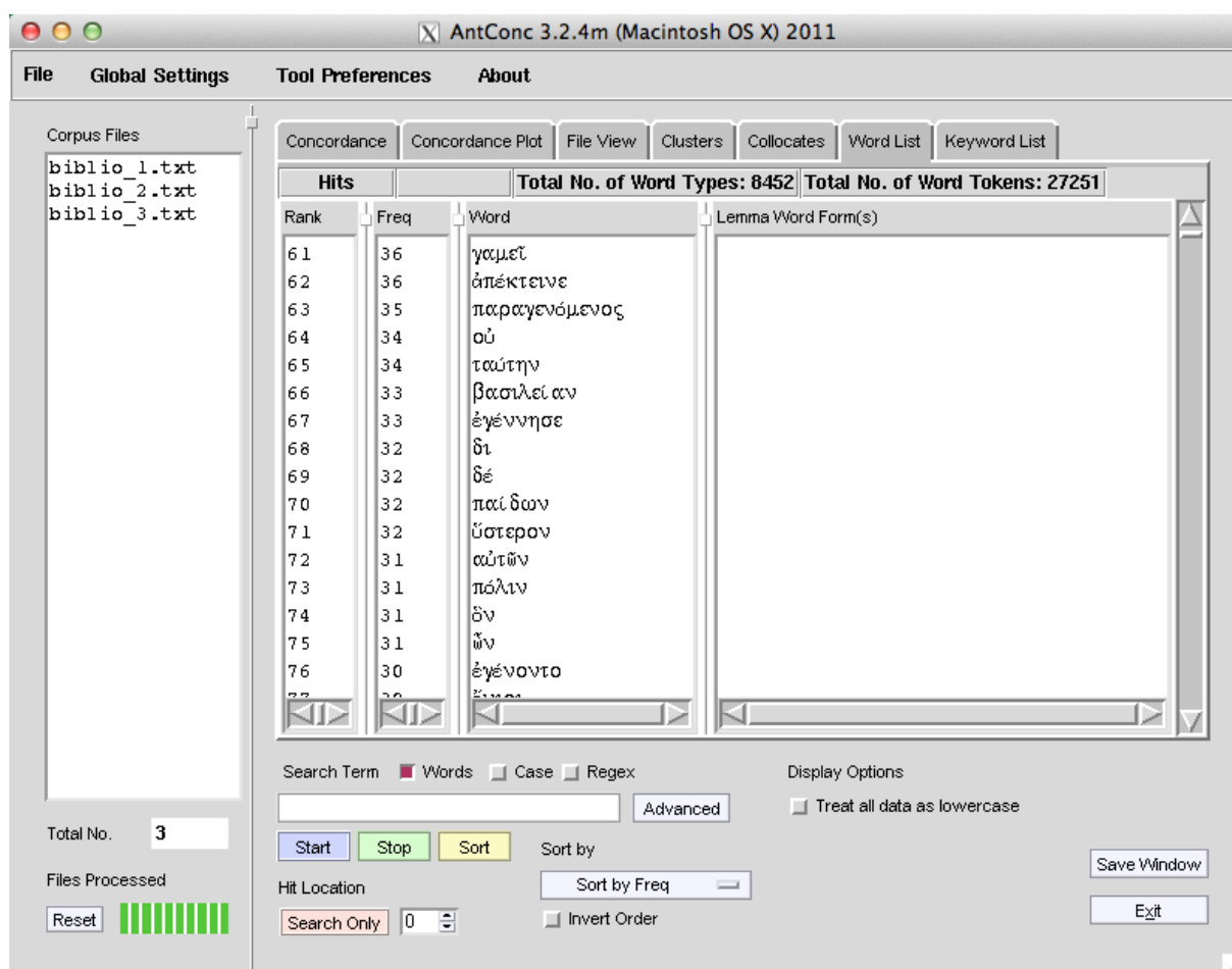
Figura 14. Tela da função Word List (lista de palavras) do AntConc classificada por frequência
