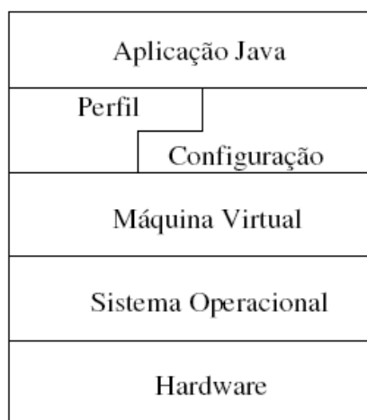
Figura 4.7 - Arquitetura J2ME.
