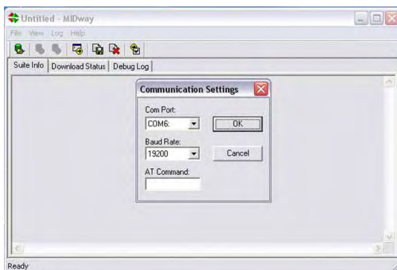
Figura C.3 - Programa MIDway 2.8.
