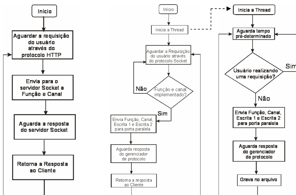
Figura 6.6 - Fluxograma da parte lógica do processador NCAP.
