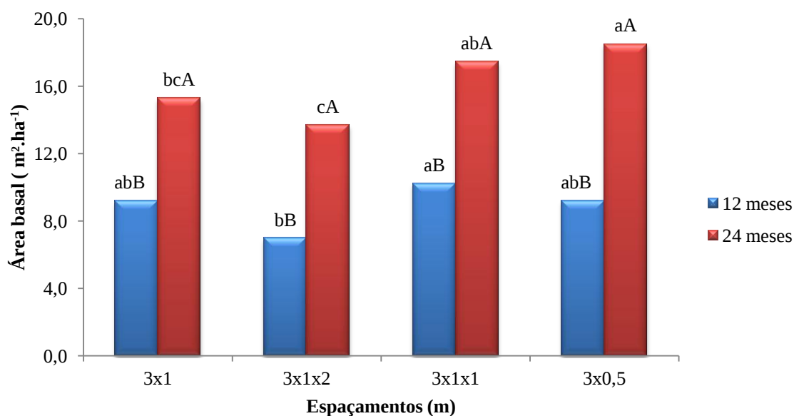
Figura 8. Área basal aos 12 e 24 meses de idade. Conforme teste de Tukey a 5% de probabilidade – letras maiúsculas entre idades e letras minúsculas entre espaçamentos iguais não diferem entre si.
