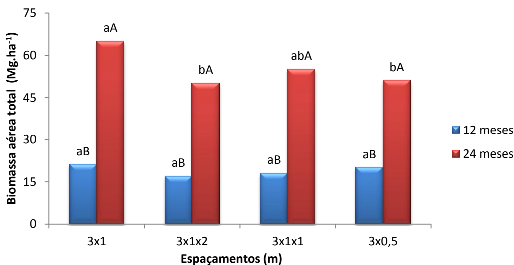
Figura 11. Biomassa aérea total aos 12 e 24 meses de idade. Conforme teste de Tukey a 5% de probabilidade – letras maiúsculas entre idades e letras minúsculas entre espaçamentos iguais não diferem entre si.
