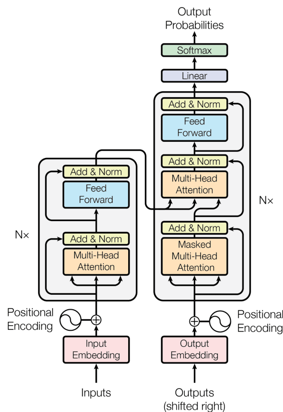
Figura 2 – Arquitetura do modelo Transformer .
