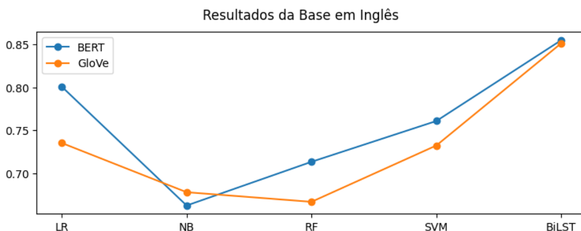
Figura 20 – Gráfico com os resultados de Sadeghi, Bidgoly e Amirkhani (2022), com o uso de premissas, na base de dados FNID-FakeNewsNet , para o conjunto de teste.
