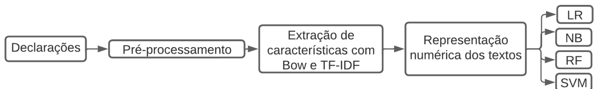
Figura 14 – Esquema dos modelos com LR, NB, RF e SVM com o uso de premissas.
