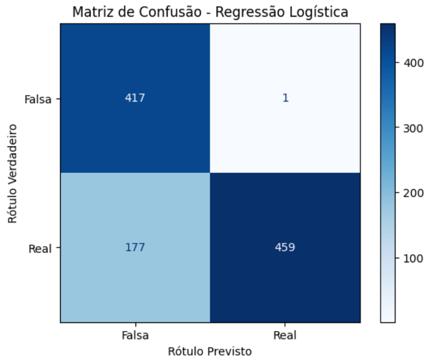
Figura 23 – Matriz de confusão da LR com premissas.
