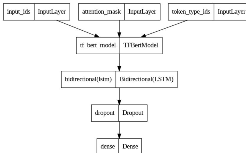
Figura 16 – Arquitetura dos modelos criados com os embeddings do BERTimbau.
