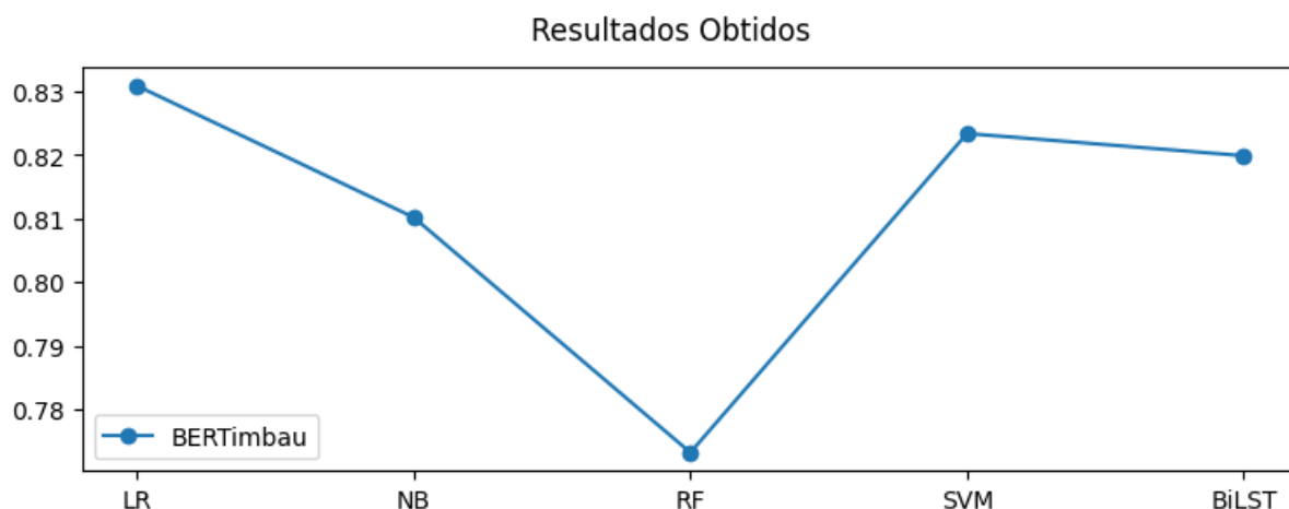
Figura 22 – Gráfico com os resultados obtidos com o método proposto, com o uso de premissas, na base de dados FNID-FakeNewsNet traduzida, para o conjunto de teste.
