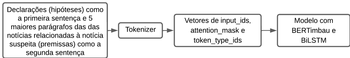
Figura 18 – Esquema do modelo com BERTimbau e BiLSTM com o uso de premissas.
