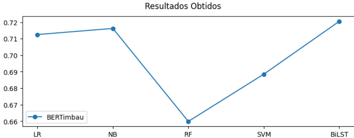
Figura 21 – Gráfico com os resultados obtidos com o método proposto, sem o uso de premissas, na base de dados FNID-FakeNewsNet traduzida, para o conjunto de teste.
