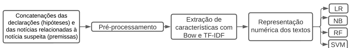
Figura 15 – Esquema dos modelos com LR, NB, RF e SVM com o uso de premissas.
