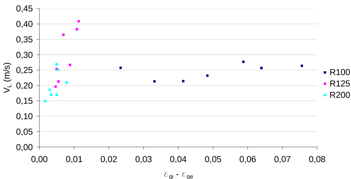
Figura 6.21: Velocidade de circulação do líquido em função da diferença entre \varepsilon_{gi} e \varepsilon_{ge} para os reatores R100, R125 e R200
