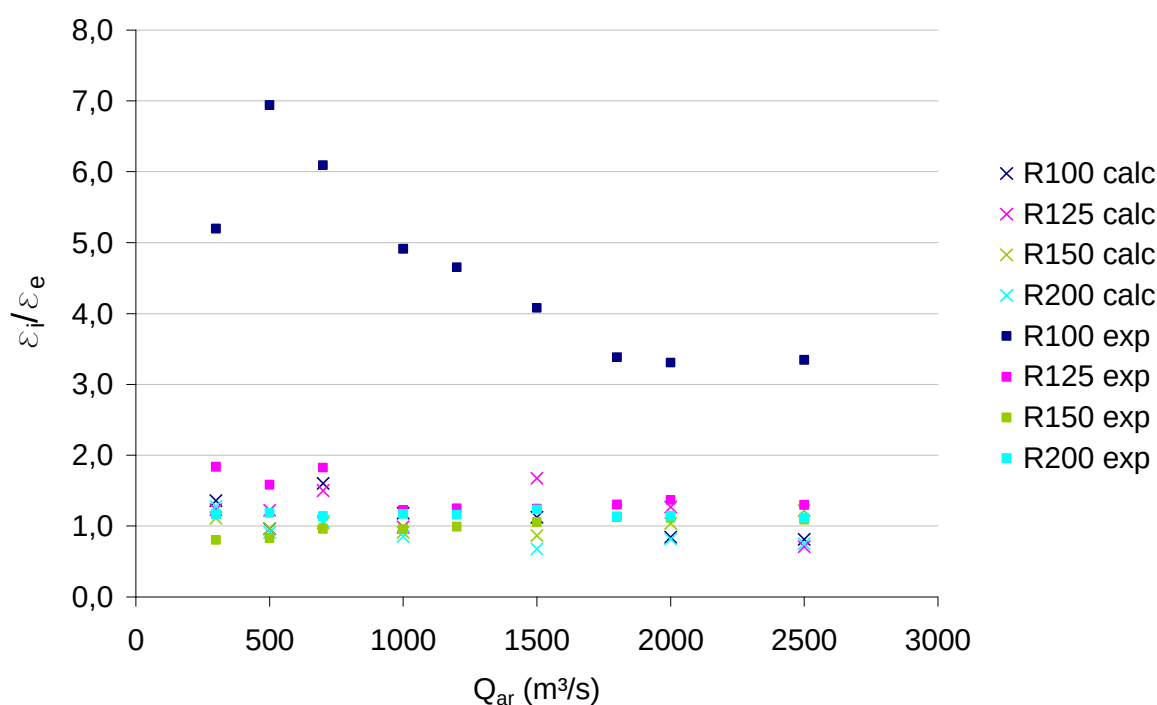
Figura 6.23: Razão entre \epsilon_i e \epsilon_e calculadas pela equação da continuidade e medidas experimentalmente em função da vazão de ar injetada no sistema
