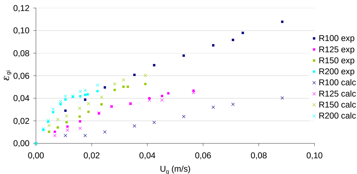
Figura 6.14: Comparação entre a fração volumétrica de ar experimental e a calculada pela relação de Lu et al. (1995) para o tubo interno em meio bifásico
