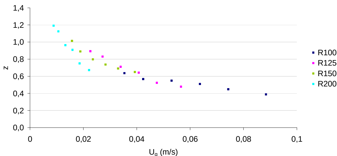
Figura 6.3: Valores de z em função da velocidade superficial do gás obtidos para meio bifásico
