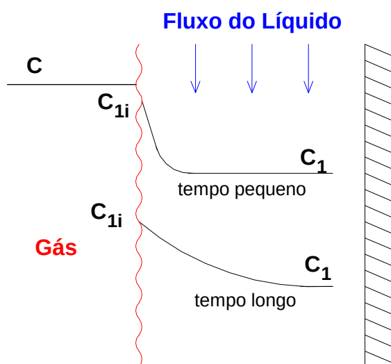
Figura 4.12: Representação esquemática da Teoria da Penetração. Adaptado de Cussler (1997)
