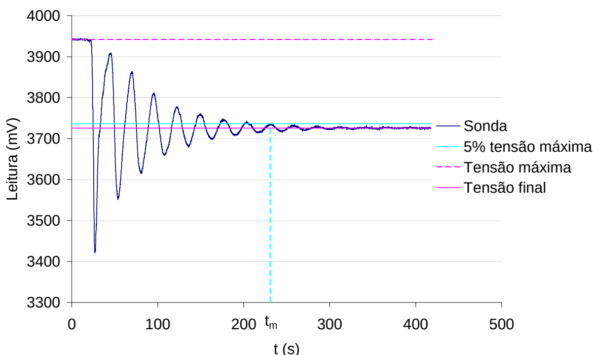
Figura 5.10: Exemplo de procedimento para determinação do tempo de mistura
