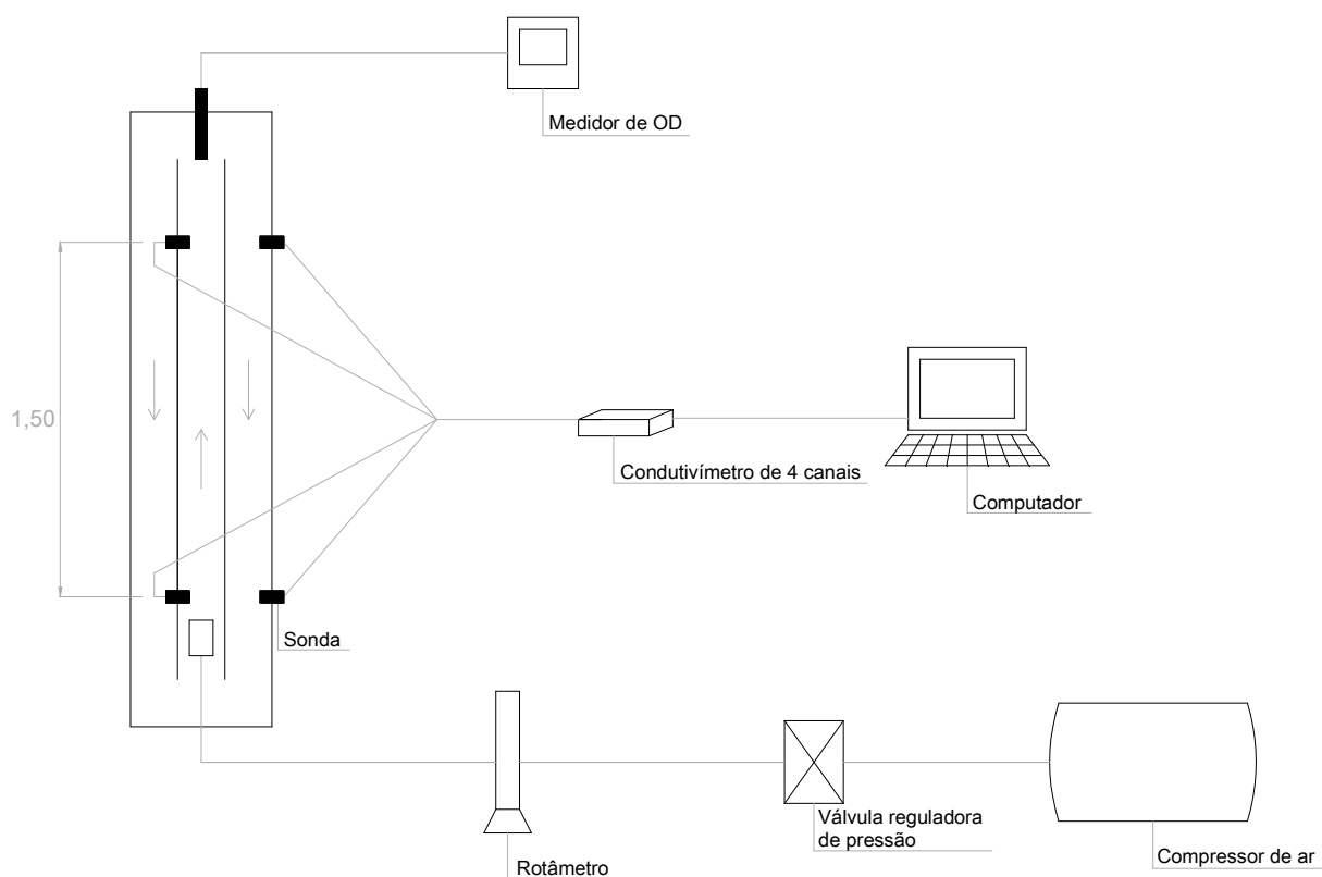
Figura 5.6: Representação esquemática dos equipamentos utilizados.
