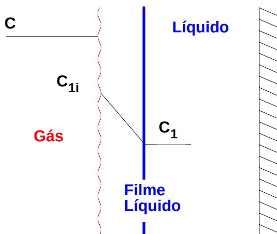
Figura 4.11: Representação esquemática da Teoria do Filme. Adaptado de Cussler (1997)
