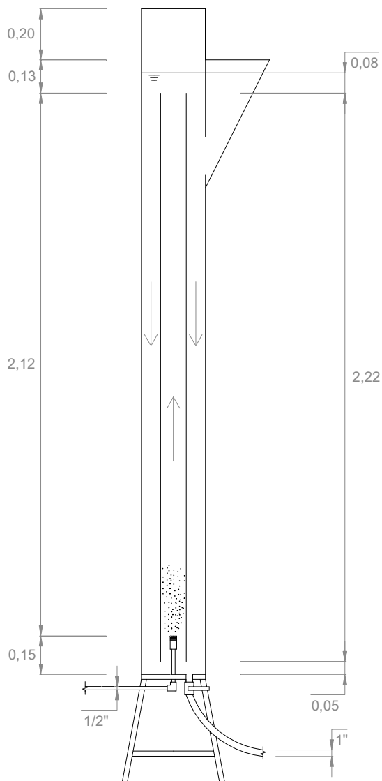
CORTE AA'
