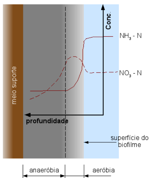
Figura 4.20: Perfil de nitrogênio no interior do biofilme. Adaptado de Iwai e Kitao (1994) por Gebara (2006)
