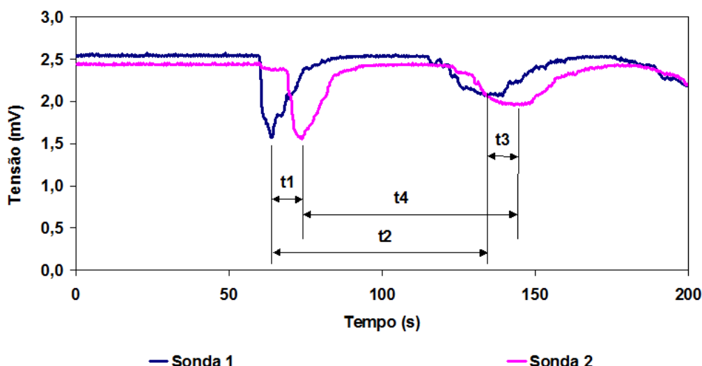
Figura 5.9: Tensão em função do tempo durante ensaio com traçador
