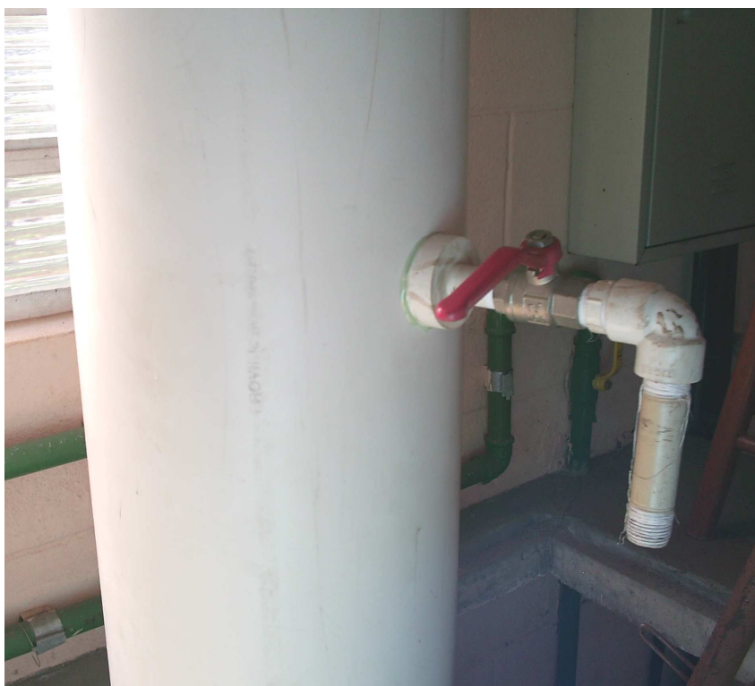
Figura 5.7: Detalhe da torneira para retirada de amostra do reator
