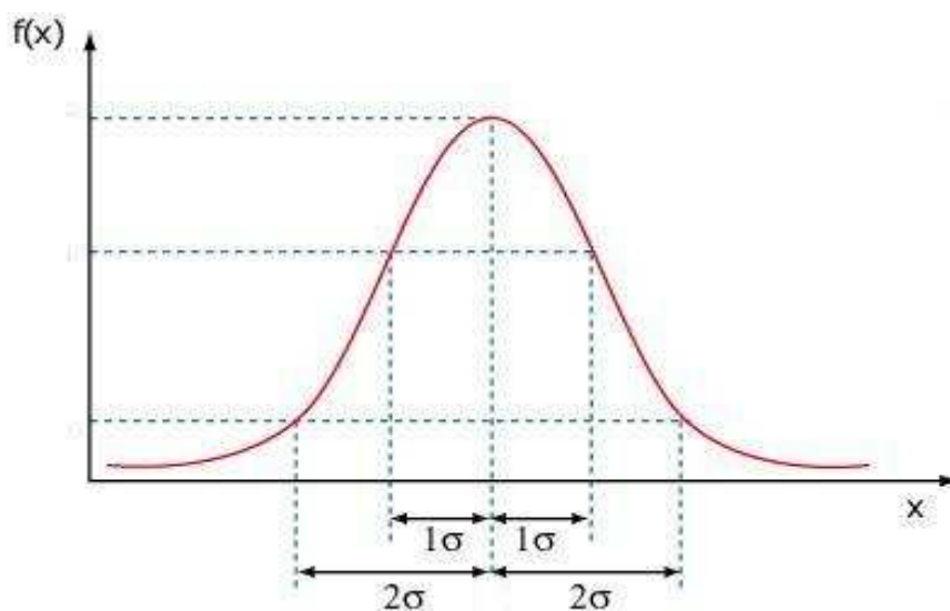
Figura 5.11: Distribuição normal na Curva de Gauss
