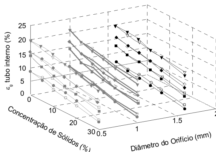
Figura 4.6: Influência da concentração e massa específica dos sólidos sobre a fração volumétrica de gás em função do diâmetro do orifício do injetor e da vazão de ar (2100 l/h: O - BME, ● - AME; 5300 l/h: □ - BME, ■ - AME; 8000 l/h: ◇ - BME, ◆ - AME; 11800 l/h: ▽ - BME, ▼ - AME); BME – baixa massa específica; AME – alta massa específica. Adaptado de Freitas et al. (2000)
