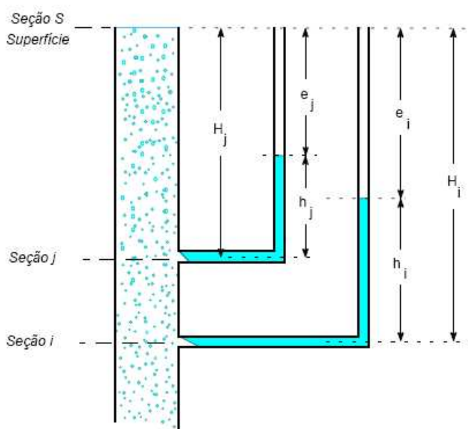
Figura 5.13: Esquema para cálculo da expansão do leito Fonte: (DALL'AGLIO SOBRINHO et al., 2000)
