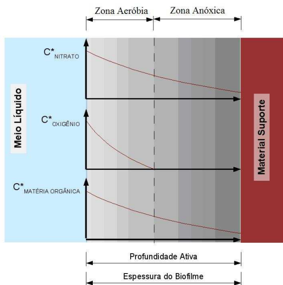
Figura 4.18: Perfil de concentração de oxigênio, matéria orgânica e nitrato no biofilme – Completamente penetrado pelo nitrato. Adaptado de Hagedorn-Olsen et al. (1994) por Gebara (2006)
