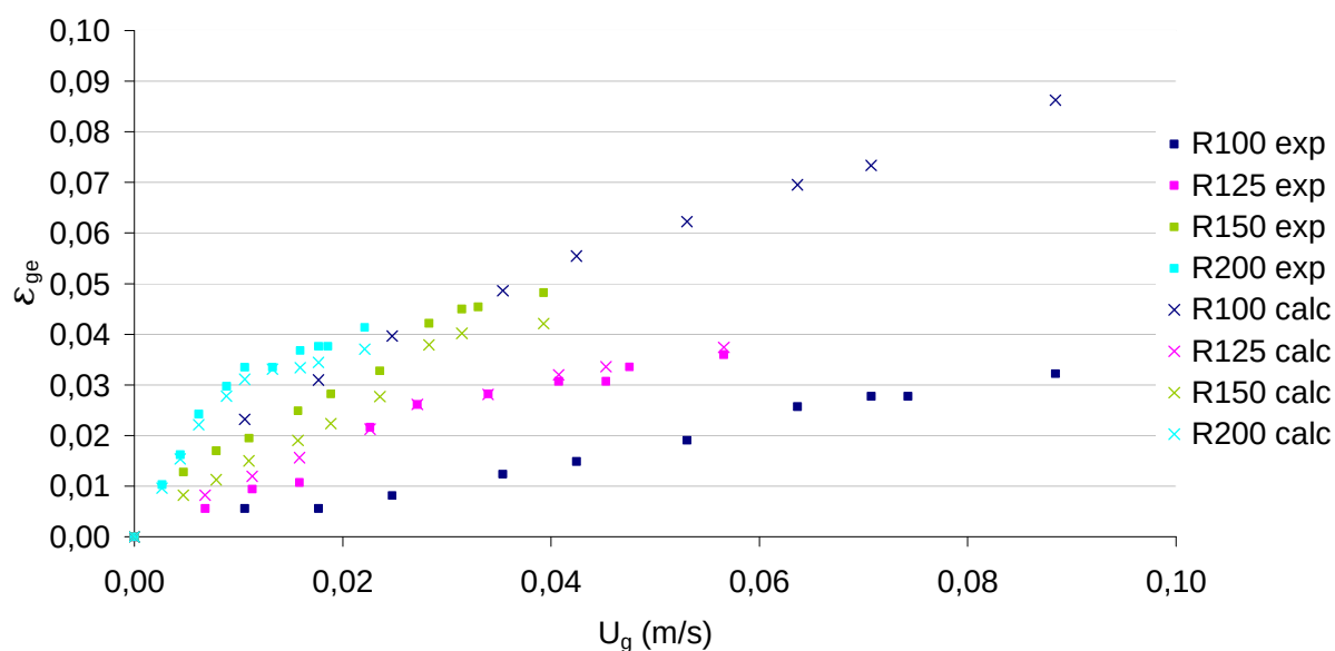
Figura 6.15: Comparação entre a fração volumétrica de ar experimental e a calculada pela relação de Lu et al. (1995) para o tubo externo em meio bifásico
