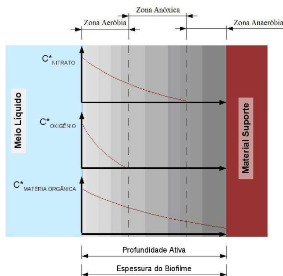
Figura 4.19: Perfil de concentração de oxigênio, matéria orgânica e nitrato no biofilme – Parcialmente penetrado pelo nitrato. Adaptado de Hagedorn-Olsen et al. (1994) por Gebara (2006)
