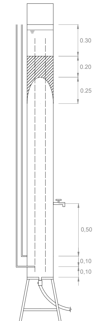
CORTE BB'
