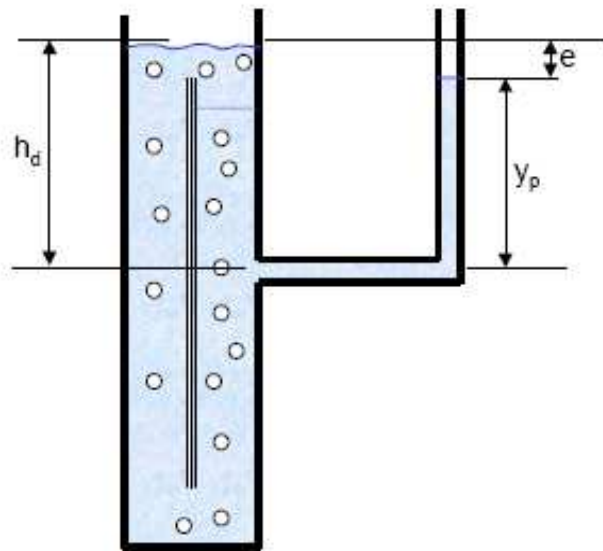
Figura 5.14: Esquema para cálculo da fração volumétrica de ar Fonte: (RUGGERI JÚNIOR, 2002)
