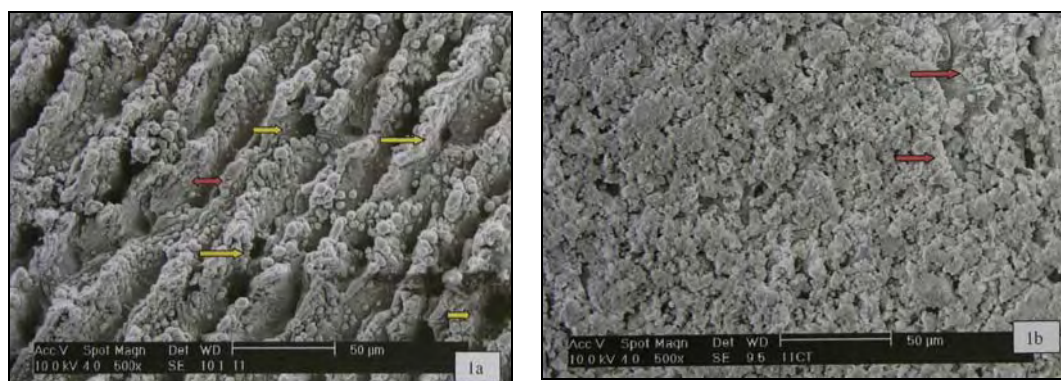
Figura 1 – 1a – Fotomicrografia mostrando o disco tratado com Laser em aumento de 500x sob MEV. Notam-se zonas de fusão e solidificação rápidas resultando na presença de defeitos lineares com aproximadamente 25µm de espessura (Seta vermelha) e presença de poros na superfície (Setas amarelas). (SISTI, 2004) 31
