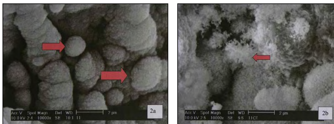
Figura 2 – 2a – Fotomicrografia do disco tratado com laser em aumento de 10.000x sob MEV, evidenciando a presença de esferas com rugosidade superficial e textura áspera (Setas vermelhas). (SISTI, 2004) 31
