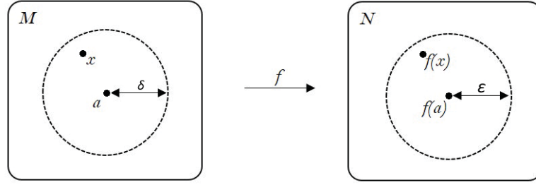
Figura 6.1: Continuidade em espaços métricos.
