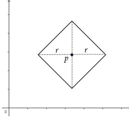
Figura 4.12: Esfera no \mathbb{R}^2 usando a métrica d_1 .
