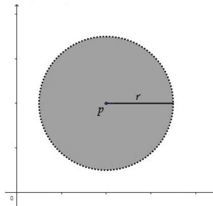
Figura 4.7: Bola aberta no \mathbb{R}^2 usando a métrica d .
