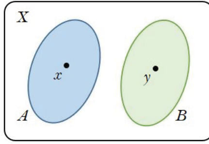
Figura 5.3: Pontos x \neq y em um Espaço de Hausdorff. Fonte: Elaborada pela autora.
