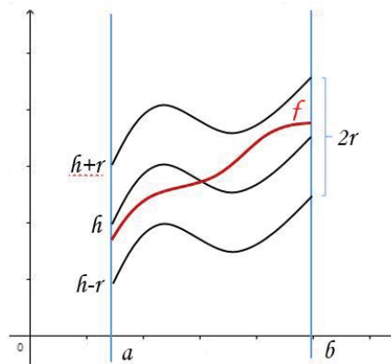
Figura 4.17: Bola fechada no \mathcal{C}[a, b] usando a métrica do supremo.
