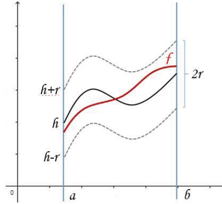
Figura 4.16: Bola aberta no \mathcal{C}[a, b] usando a métrica do supremo.
