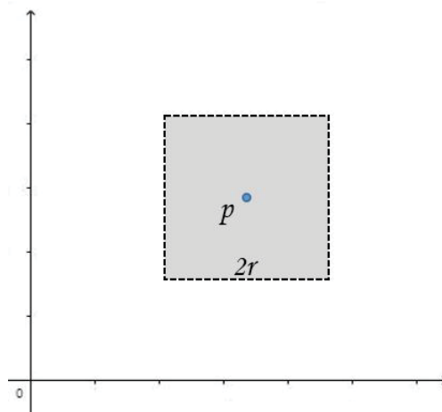
Figura 4.13: Bola aberta no \mathbb{R}^2 usando a métrica d_2 .
