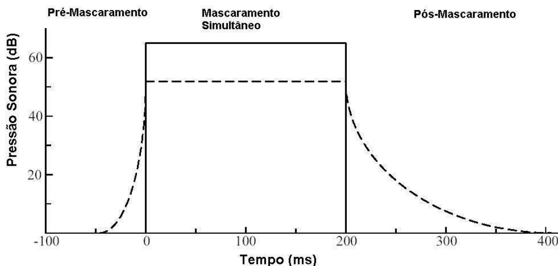
Figura 10 – Principais tipos de mascaramento (CAVE, 2002).
