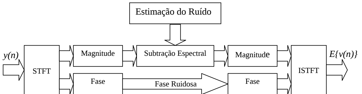
Figura 17 – Esquema básico da subtração espectral.
