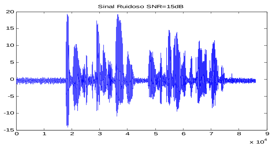
Figura 31 – Forma de onda do sinal 1 com SNR = 15dB.
