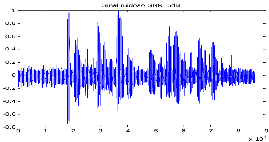
Figura 29 – Forma de onda do sinal 1 com SNR = 5dB.
