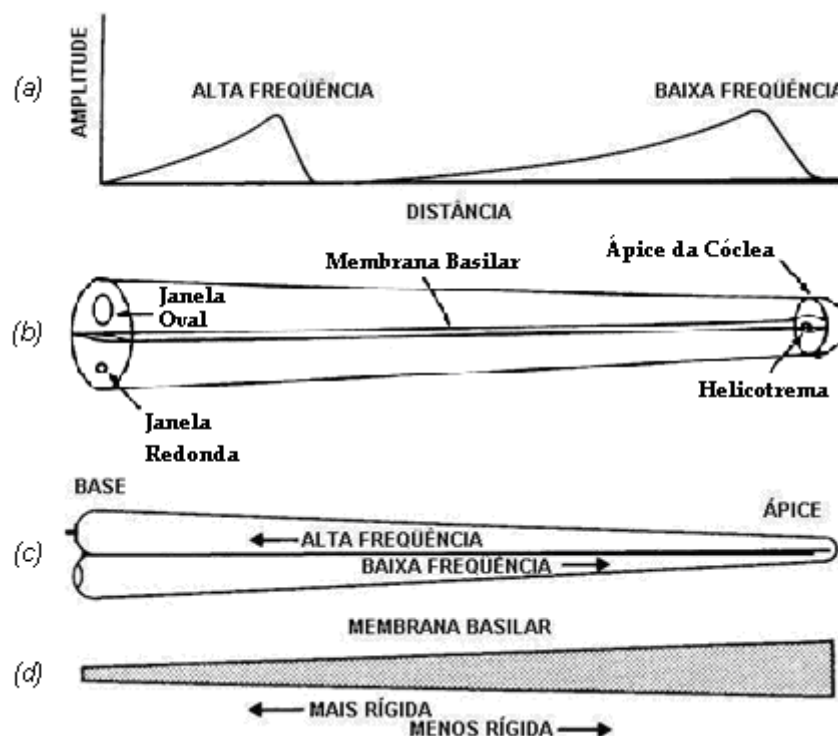
Figura 5 – Propriedades da membrana basilar, (a) amplitude da vibração da membrana basilar em função da distância de sua base, (b) componentes de sua estrutura, (c) relação entre a frequência do sinal e a posição da oscilação ao longo da membrana, (d) relação entre a rigidez da membrana em função da distância da base (LEITE, 2003).
