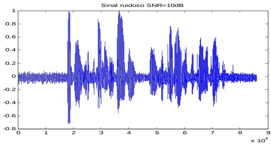
Figura 30 – Forma de onda do sinal 1 com SNR = 10dB.
