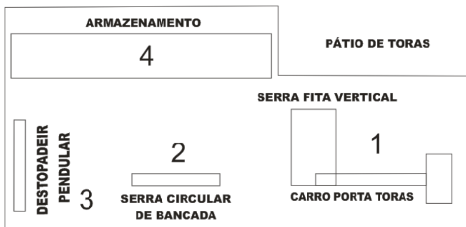
Figura 6 - Layout da serraria
