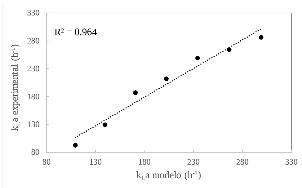
Figura 20. Valores de k_{La} ( \text{h}^{-1} ) em água 28^\circ \text{C} com aeração 5,0 \text{ L}\cdot\text{min}^{-1} obtidos experimentalmente versus valores calculados pela equação 5.
