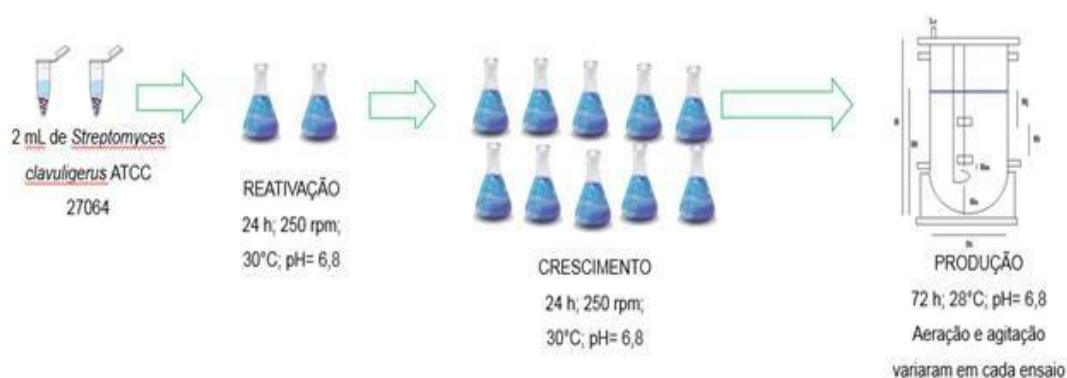
Figura 13. Procedimento experimental para produção de ácido clavulânico em biorreator com Streptomyces clavuligerus (arquivo próprio).
