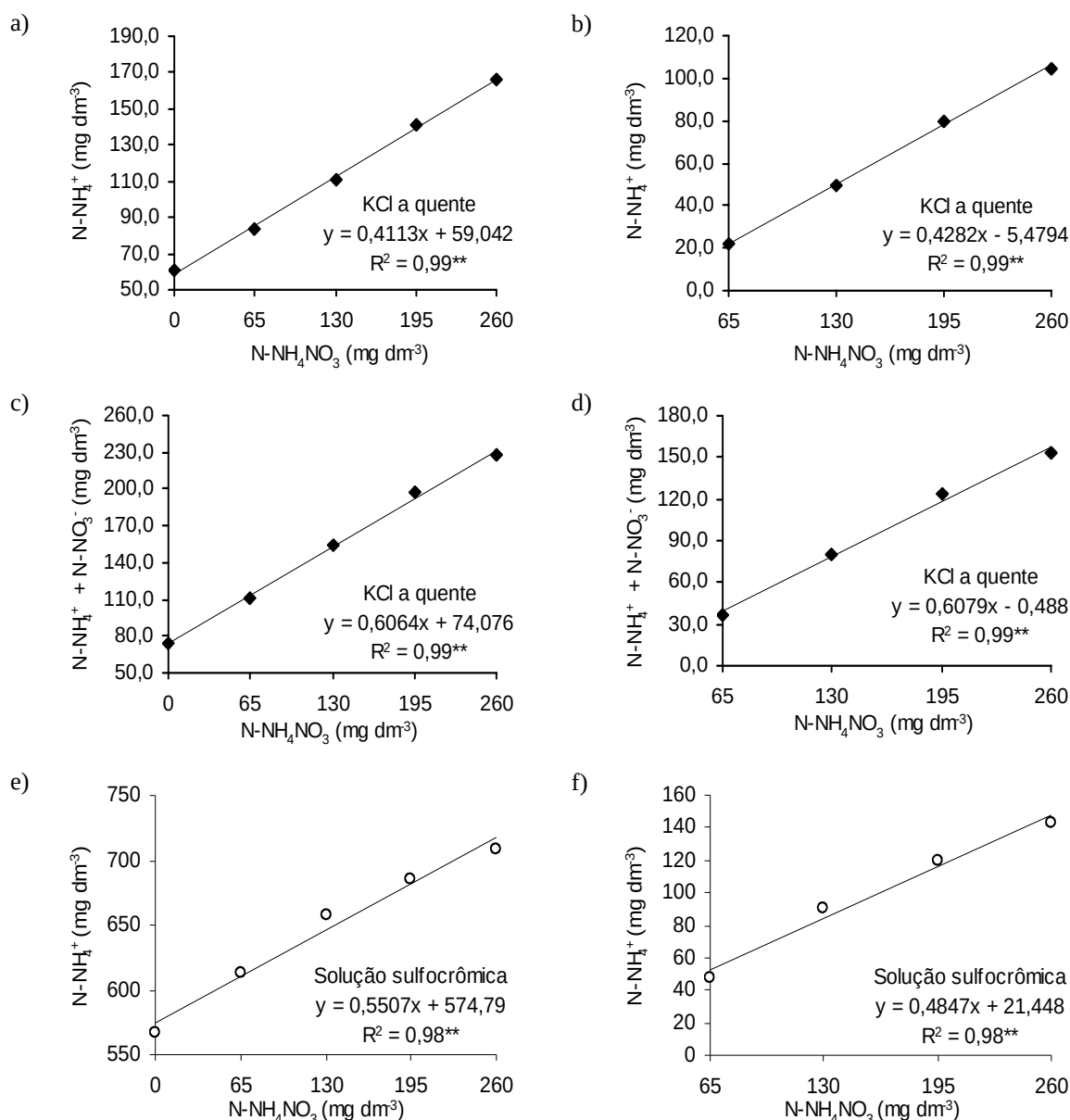
Figura 5. Teores de N-NH_4^+ ou de N-NH_4^+ + N-NO_3^- , determinados com os métodos que utilizam KCl a quente (a,b,c,d) ou solução sulfocrômica (e,f), em função de aplicação de doses de N-NH_4NO_3 , subtraindo-se (b, d e f) ou não (a, c e e) os teores de Nd do tratamento testemunha. **: significativo a 1%.
