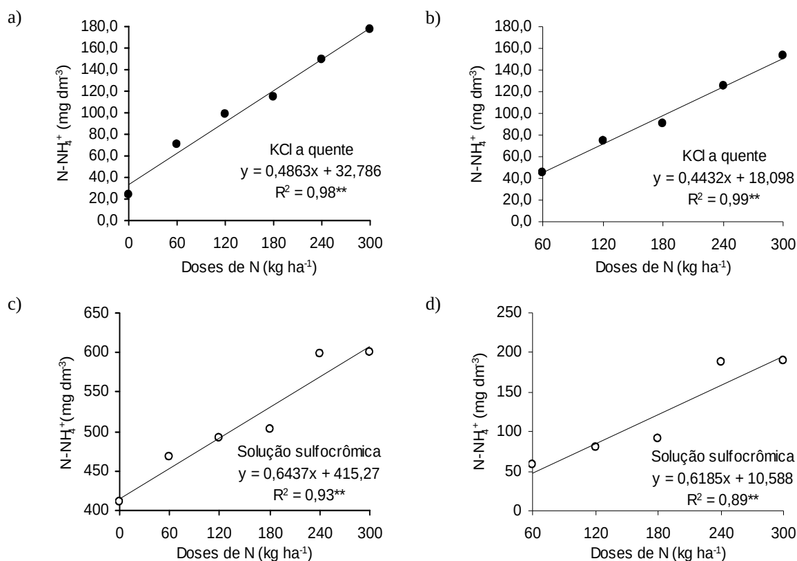
Figura 8. Teores de N-NH_4^+ determinados com os métodos que utilizam KCl a quente (a e b) ou solução sulfocrômica (c e d), em função de aplicação de doses de N, subtraindo-se (b e d) ou não (a e c) os teores de Nd do tratamento testemunha. **: significativo a 1%.
