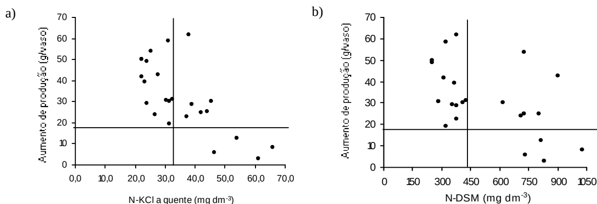
Figura 2. Níveis críticos de N disponível do solo determinados a partir de relações entre o aumento de produção de matéria seca e as extrações de N com KCl a quente (N-KCl a quente) (a) e solução sulfocrômica (N-DSM) (b).
