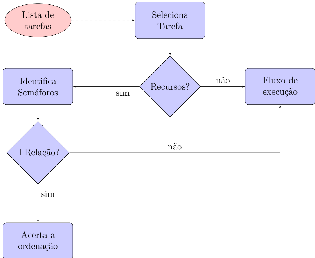
Figura 5.5: Fluxograma do escalonamento com recursos modelados
