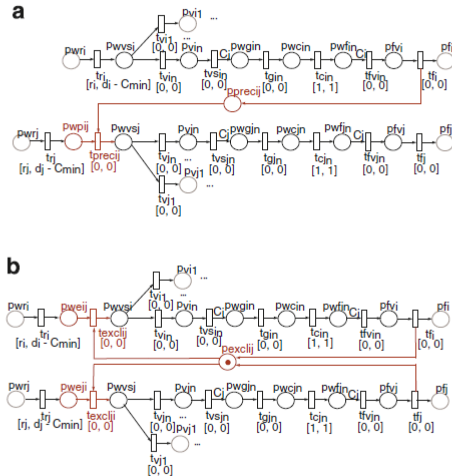
Figura 3.6: Modelos para tratamento de relações de precedência (a) e exclusão mútua (b)
