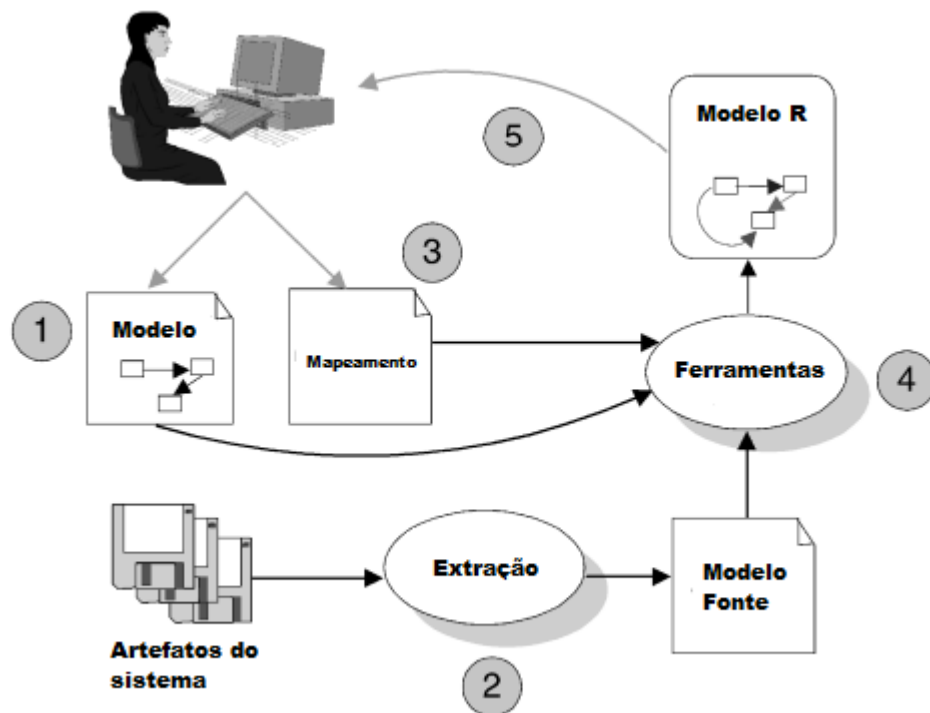
Figura 3.4: Aplicação de Software Reflexion (MURPHY; NOTKIN; SULLIVAN, 2001)
