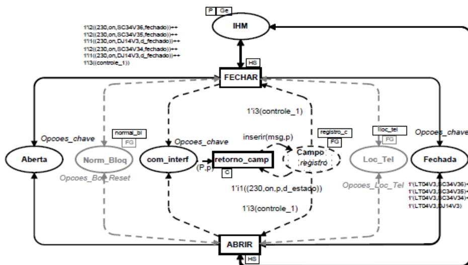
Figura 3.5: Modelo de elemento construído para o trabalho
