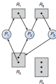
Figura 2.1: Grafo de alocação de recursos com deadlock
