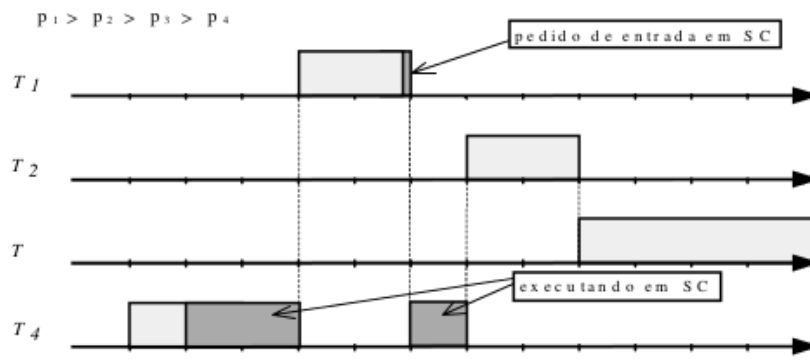
Figura 2.4: Ocorrência de inversão de prioridades
