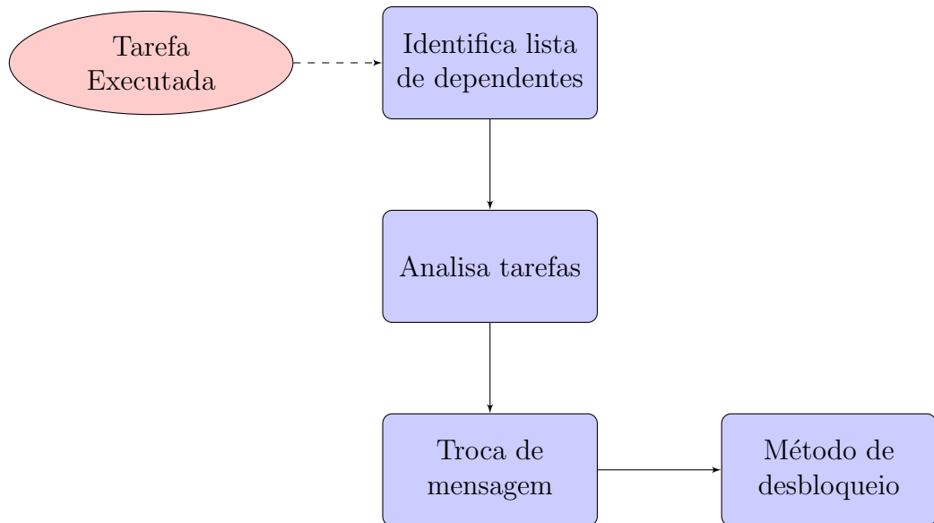
Figura 5.3: Fluxograma do tratamento de precedência com passagem de informação no modelo - Trecho de sinalização da troca
