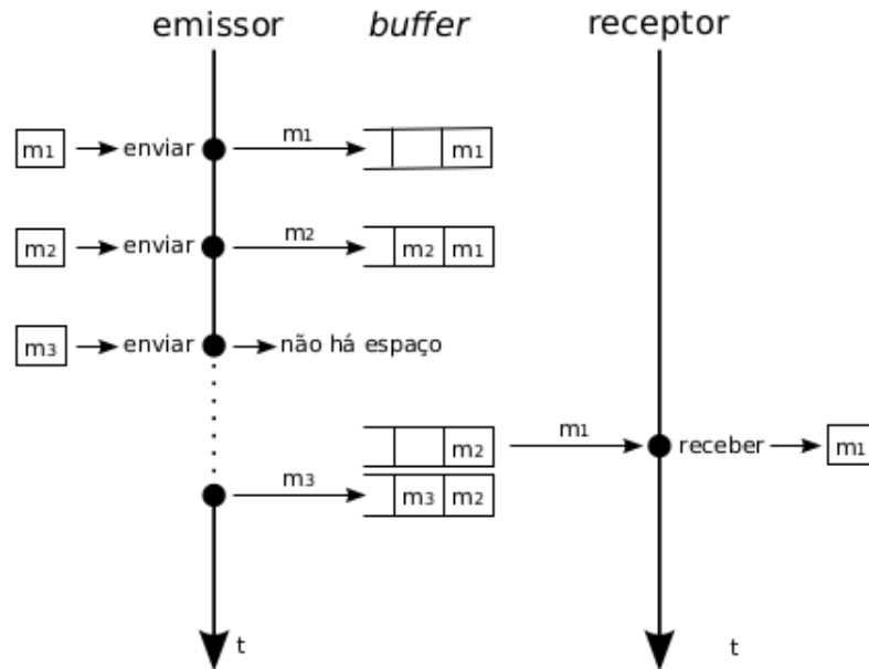
Figura 2.3: Comunicação síncrona de canal com capacidade 2
