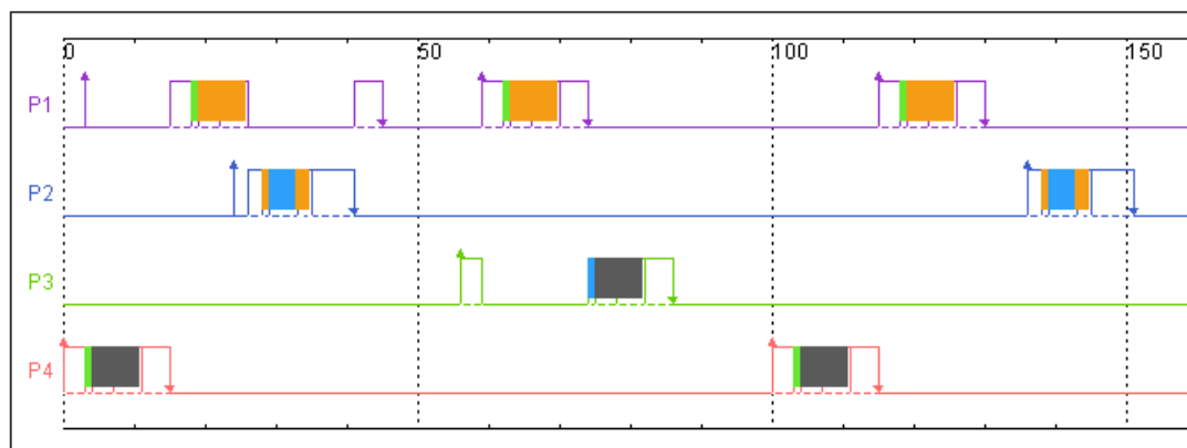
Figura 6.17: Exemplo de escalonamento para execução com recursos
