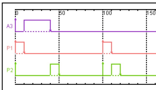
Figura 6.5: Execução no algoritmo Servidor por Deferência
