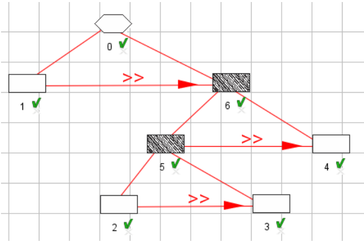
Figura 6.2: Modelo com interações de precedência entre as tarefas
