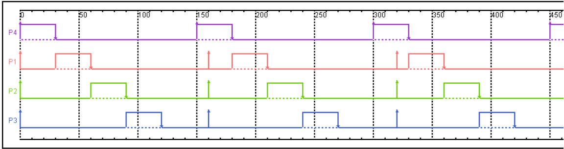
Figura 6.1: Escalonamento produzido com o algoritmo Taxa Monotônica
