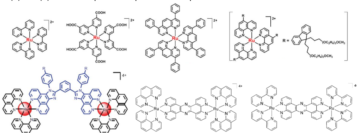
Figure 4. Structure chimique de certains complexes monomères de Ru(II) et bimétalliques Ru(II)—Ru(II) excitables par l'absorption de deux photon. 40-42
