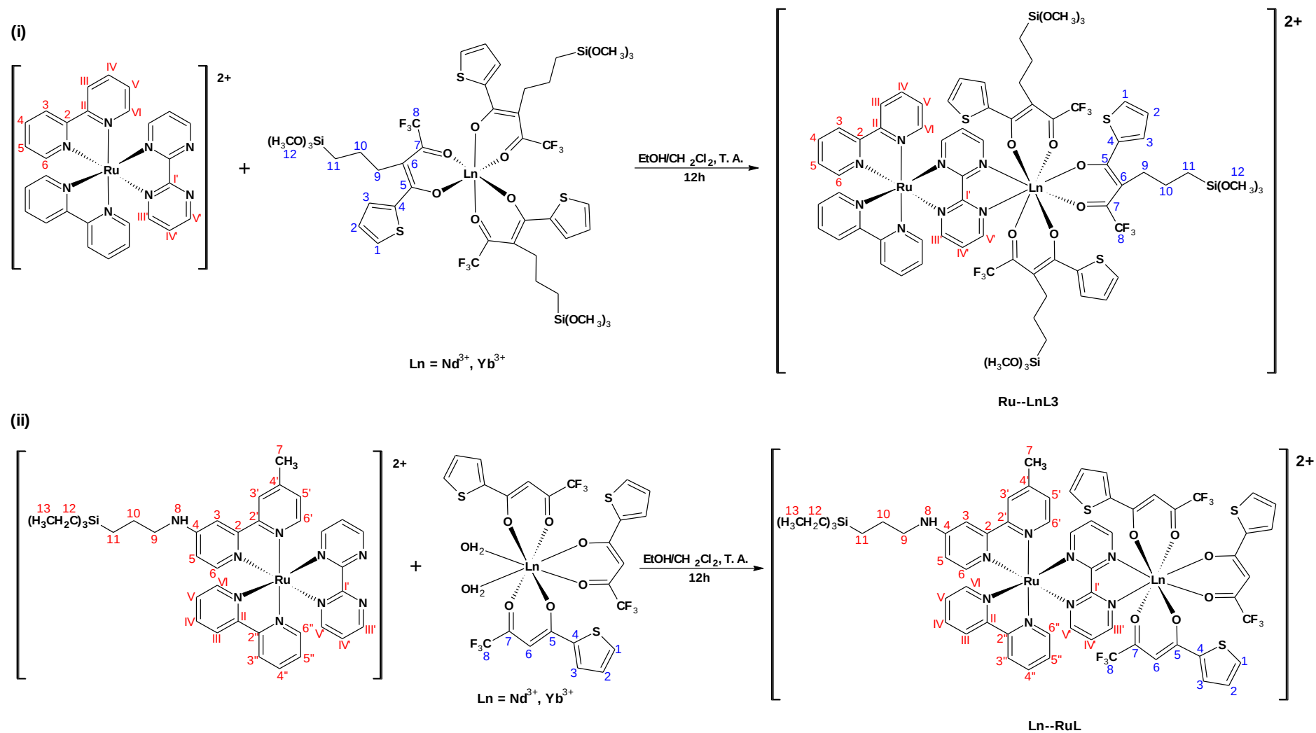
Figure 7. Voies de synthèse et structures proposées pour les complexes hétérochimériques silylés Ru—LnL3 (i) and Ln—RuL (ii), ( \text{Ln} = \text{Nd}^{3+}, \text{Yb}^{3+} ).
