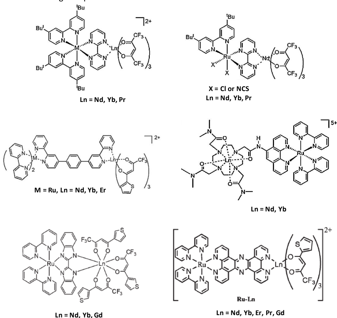
La figure 5. Exemples représentatifs de complexes hétérobimétalliques d-f (Ru—Ln) mettant en œuvre des ligands pontants décrits dans la littérature. 13, 22, 28, 29
