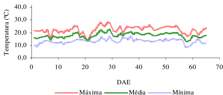
Figura 6. Temperatura do ar máxima, média e mínima no interior do ambiente protegido, durante a condução da cultura (maio a julho de 2006).
