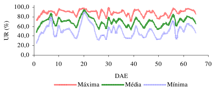
Figura 7. Umidade relativa do ar máxima, média e mínima no interior do ambiente protegido, durante a condução da cultura (maio a julho de 2006).
