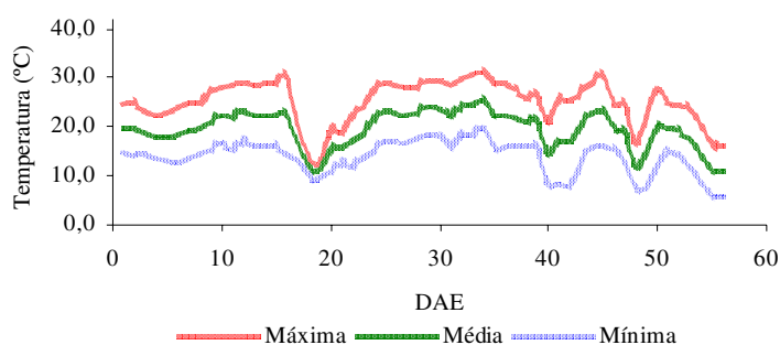
Figura 28. Temperatura do ar máxima, média e mínima no interior do ambiente protegido, durante a condução da cultura (julho a setembro de 2006).
