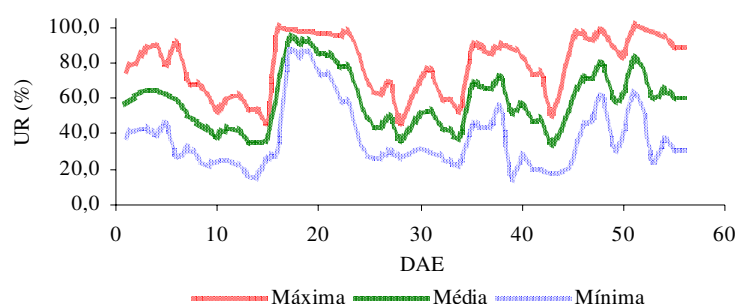
Figura 29. Umidade relativa do ar máxima, média e mínima no interior do ambiente protegido, durante a condução da cultura (julho a setembro de 2006).
