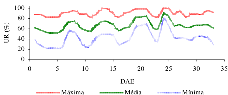
Figura 5. Umidade relativa do ar máxima, média e mínima no interior do ambiente protegido, durante a condução da cultura (novembro a dezembro de 2005).
