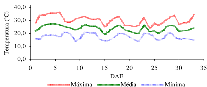
Figura 4. Temperatura do ar máxima, média e mínima no interior do ambiente protegido, durante a condução da cultura (novembro a dezembro de 2005).
