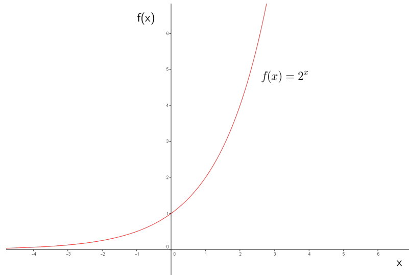
Figura 4.2: Gráfico de f(x) = 2^x
