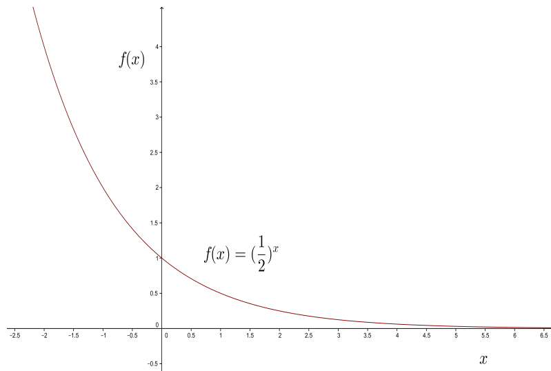
Figura 4.1: Gráfico de f(x) = \left(\frac{1}{2}\right)^x
