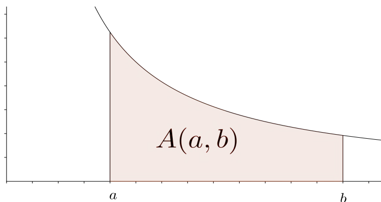
Figura 5.1: Área da região compreendida entre as retas x = a , x = b e a hipérbole y = \frac{1}{x}
