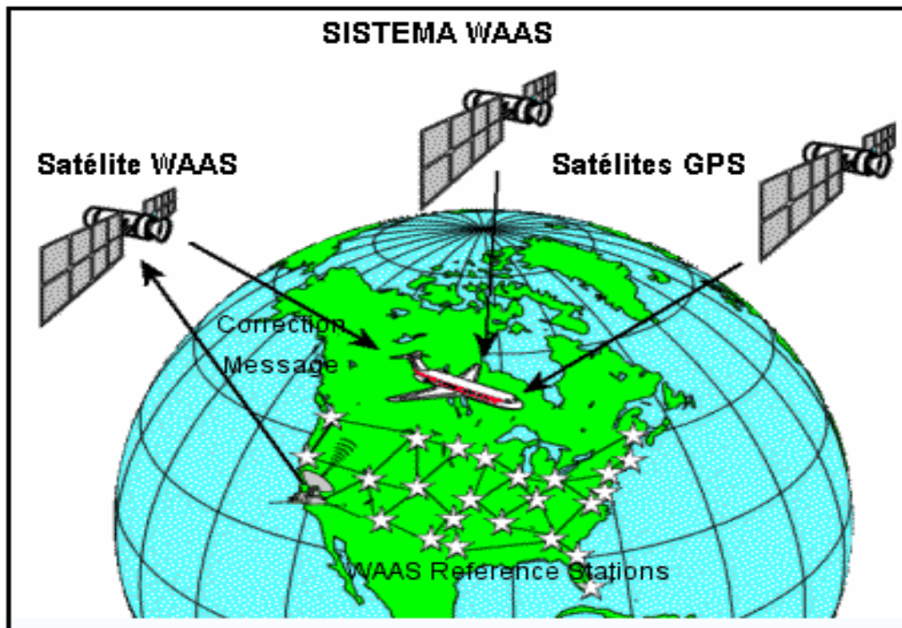
Figura 5. Sistema WAAS. Fonte: http://iono.jpl.nasa.gov/waas.html (2006) (modificado).
