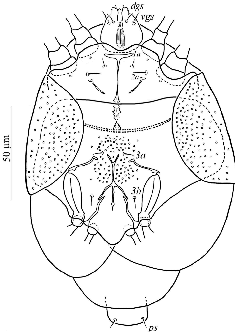
Figure 3. Excelsotarsonemus cabrucae sp. n. (female). Ventral surface.
