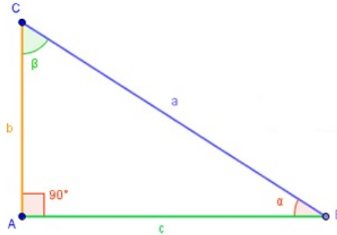
Figura 1.4: Triângulo retângulo
