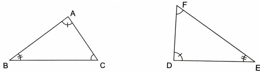
Figura 2.10: Triângulos congruentes
