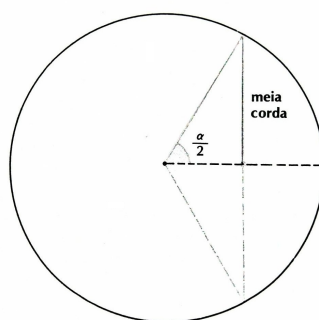
Figura 1.24: Meia corda
