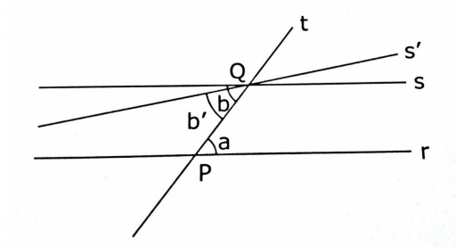
Figura 2.3: Retas paralelas
