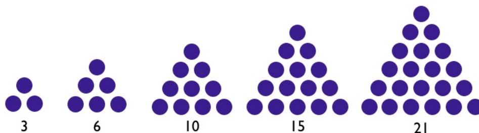
Figura 1.2: Números triangulares
