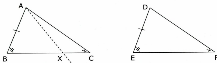
Figura 2.20: Caso LAA
