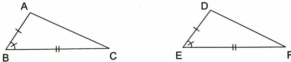
Figura 2.11: Congruência LAL
