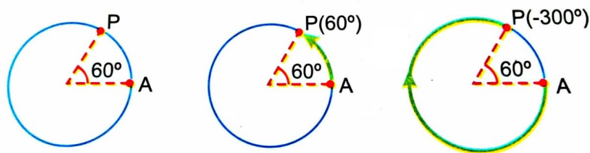
Figura 2.39: Sentidos
