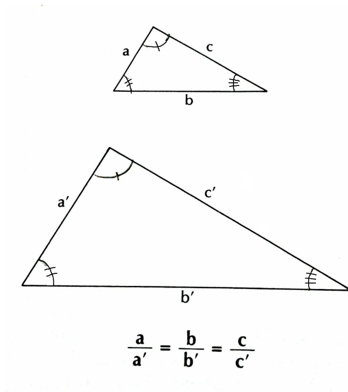
Figura 1.1: Triângulos semelhantes
