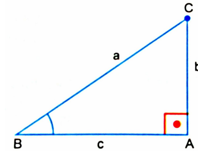
Figura 2.33: Relação fundamental
