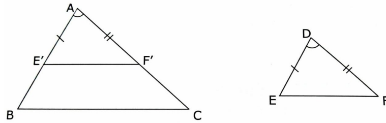
Figura 2.23: Semelhança AAA
