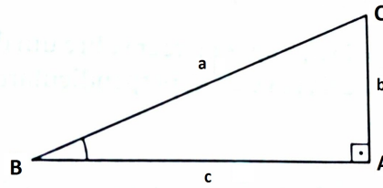
Figura 2.32: Triângulo retângulo
