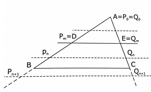
Figura 2.7: Retas paralelas
