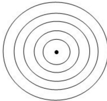
Figura 1.10: Circunferências concêntricas
