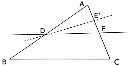
Figura 2.8: Recíproca
