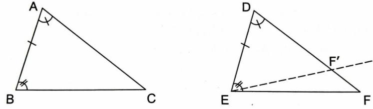
Figura 2.14: Caso ALA
