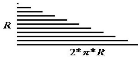
Figura 1.11: Circunferências retificadas
