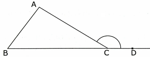
Figura 2.18: Ângulo externo
