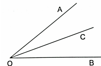
Figura 2.13: Bissetriz
