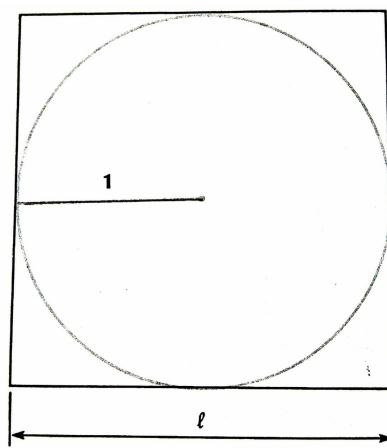
Figura 1.12: Quadrado circunscrito
