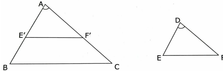
Figura 2.24: Semelhança LAL
