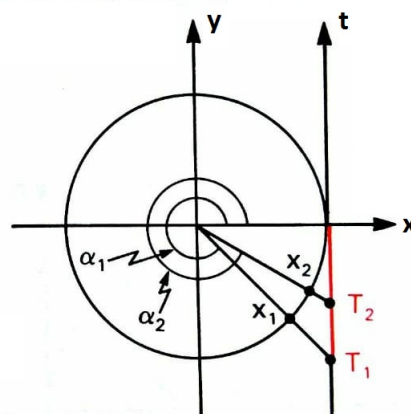
Quarto quadrante
