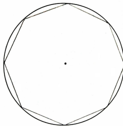
Figura 1.14: Octógono inscrito
