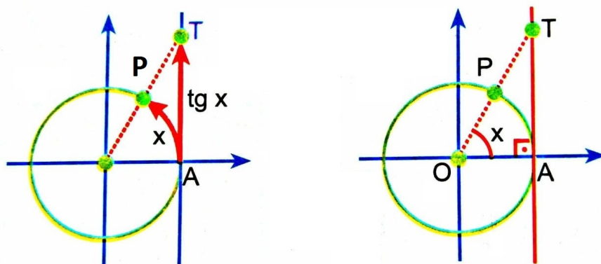
Figura 2.60: Tangentes
