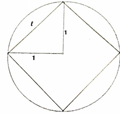
Figura 1.13: Quadrado inscrito
