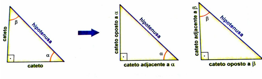
Figura 2.30: Razões trigonométricas
