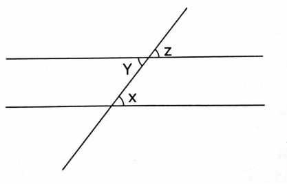
Figura 2.2: Ângulos correspondentes
