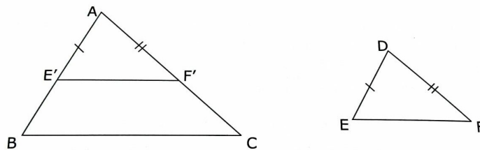
Figura 2.25: Semelhança LLL
