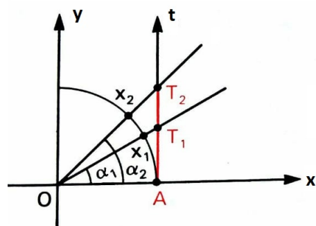
Primeiro quadrante
