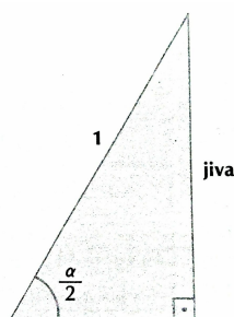
Figura 1.26: Jiva
