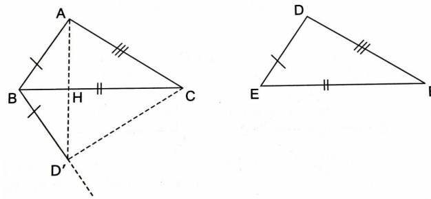
Figura 2.15: Caso LLL
