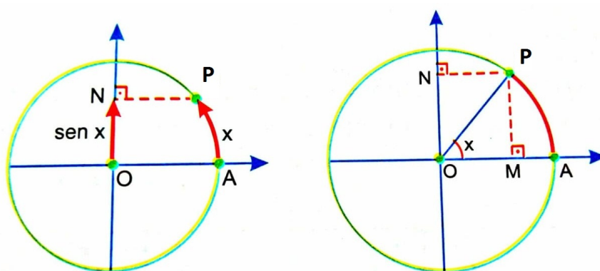
Figura 2.42: O seno
