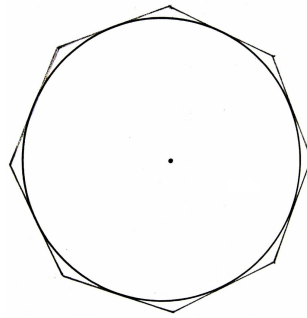
Figura 1.15: Octógono circunscrito
