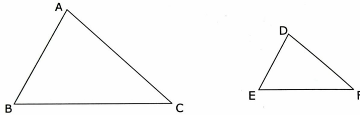
Figura 2.22: Triângulos semelhantes
