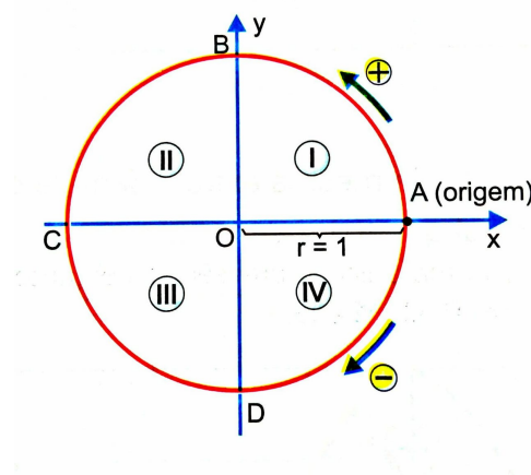
Figura 2.40: Função seno
