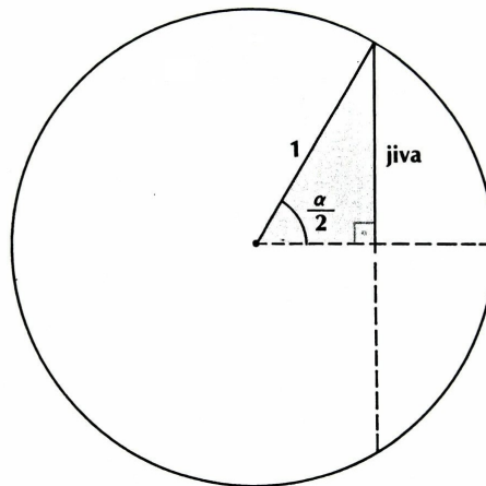
Figura 1.27: Seno
