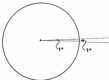
Figura 1.19: Ângulo de 1°
