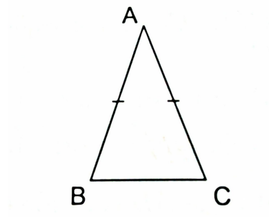
Figura 2.12: Triângulo isósceles
