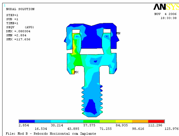
FIGURA 67 – Mapa de tensões do sistema de retenção ERA do MB.
