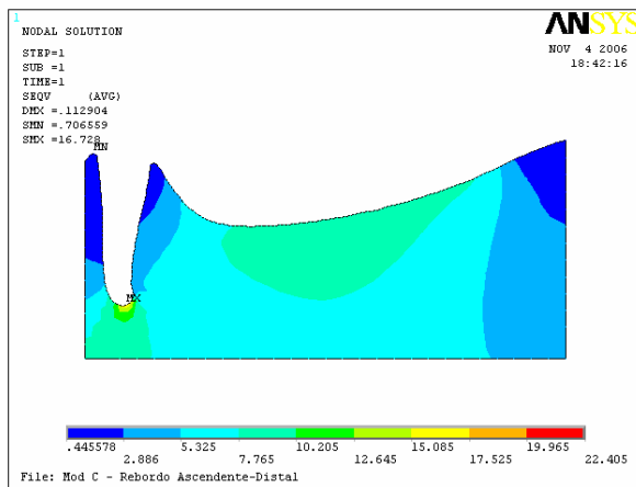
FIGURA 41 – Mapa de tensões do osso esponjoso do MC.
