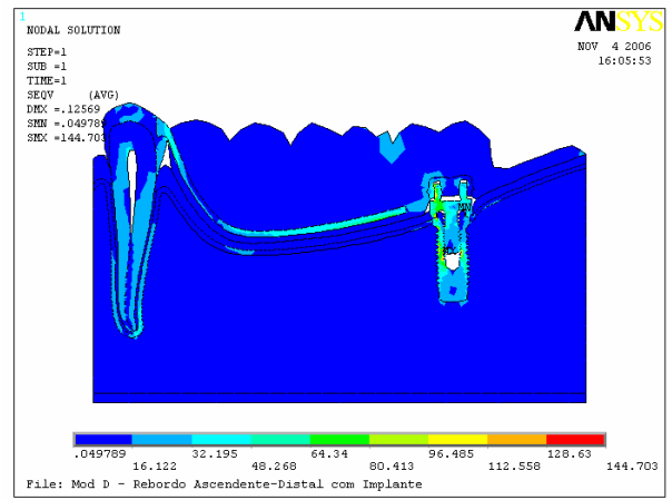
FIGURA 22 – Mapa geral da tensão de von Mises.
