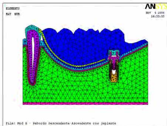
FIGURA 21 – Modelo H após a geração da malha de elementos finitos.
