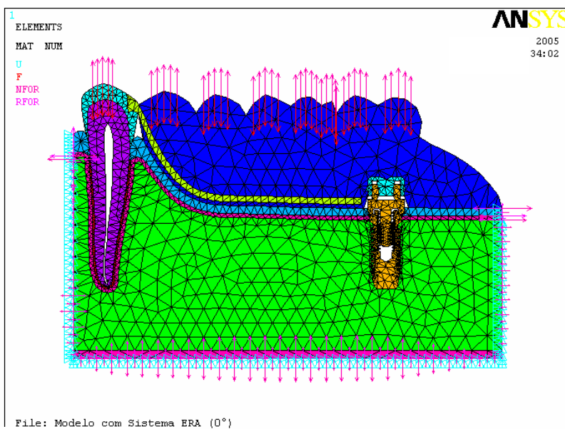
FIGURA 22 – Condições de contorno e carregamento de forças no MB.
