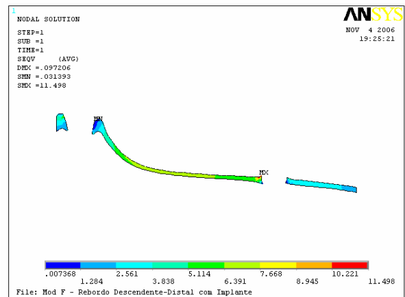
FIGURA 52 – Mapa de tensões da fibromucosa do MF.
