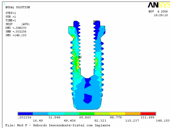
FIGURA 41 – Mapa da tensão de von Mises do implante.
