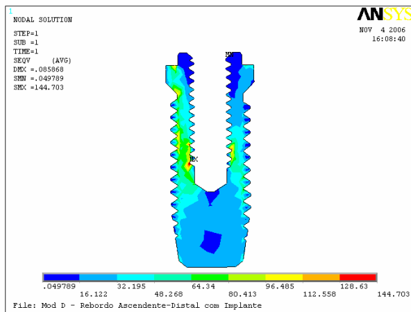
FIGURA 27 – Mapa da tensão de von Mises do implante.
