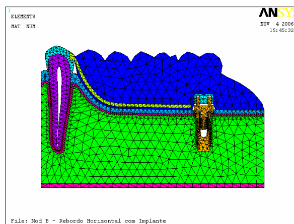
FIGURA 15 – Modelo B após a geração da malha de elementos finitos.
