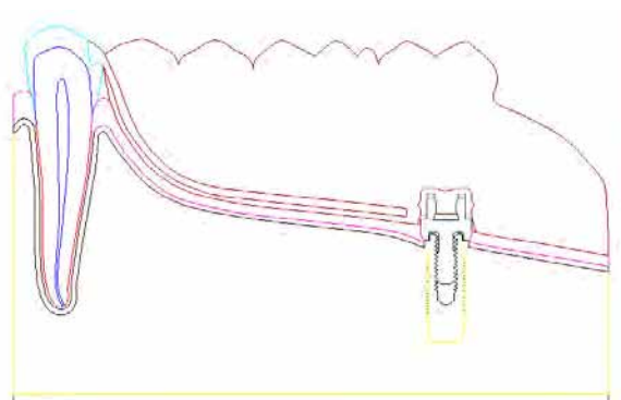
FIGURA 6 - Modelo F representando uma hemiarcadea com rebordo descendente distal, com a presença do dente 33, da PPREL e de um implante de 3,75 x 10,00 mm, com sistema ERA de retenção.
