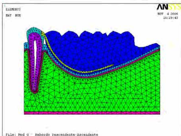
FIGURA 20 – Modelo G após a geração da malha de elementos finitos.
