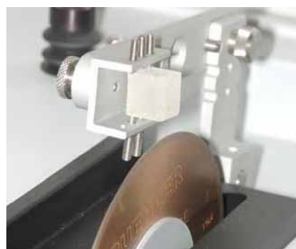
FIGURA 10 - Detalhe da superfície de corte com bloco de resina fixado.
