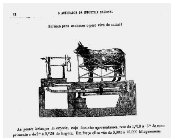
Figura 29: Desenho de balança na edição de janeiro de 1880
