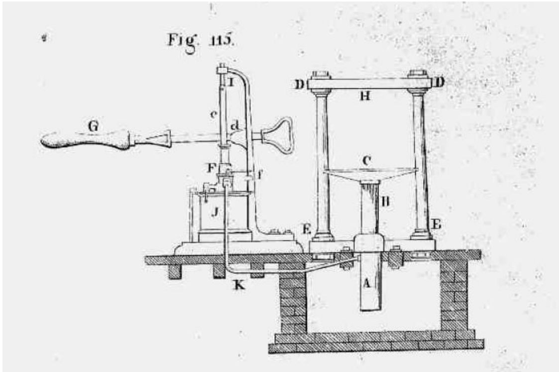
Figura 16: Prensa Hidráulica de Bramah publicada no Auxiliador da Indústria Nacional
