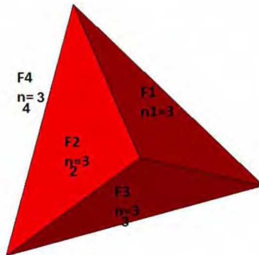
Figura 14: Faces do tetraedro.
