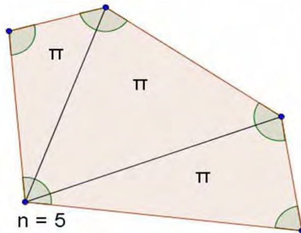
Figura 13: Soma dos ângulos internos de um pentágono.
