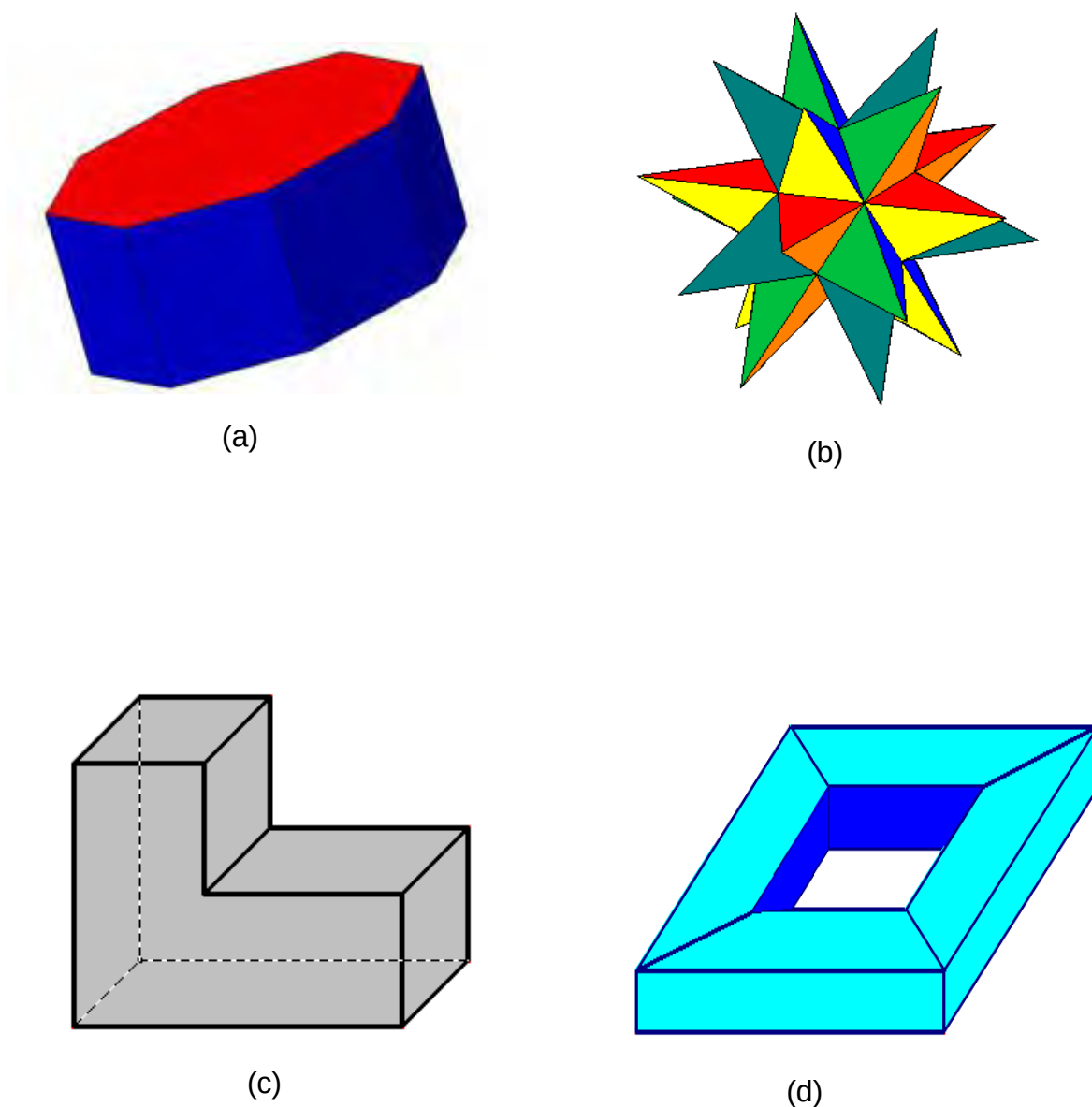
Figura 2: Exemplos de Poliedros.
