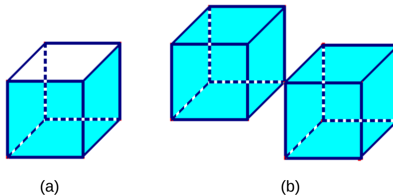
Figura 19: Exemplos de “poliedros” (definição de Cauchy).
