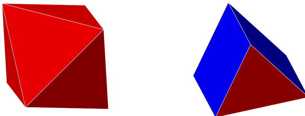
Figura 6: Exemplo de poliedro regular e não regular.
