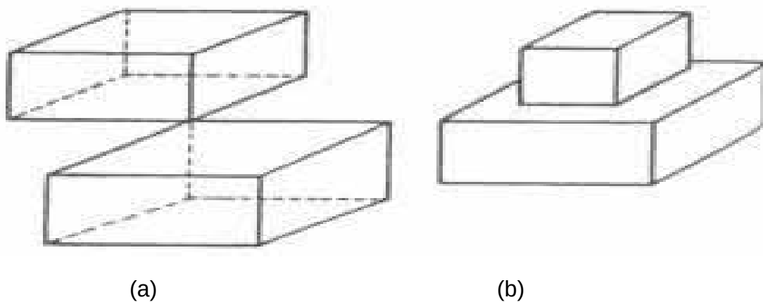
Figura 3: Exemplos de não-poliedros.
