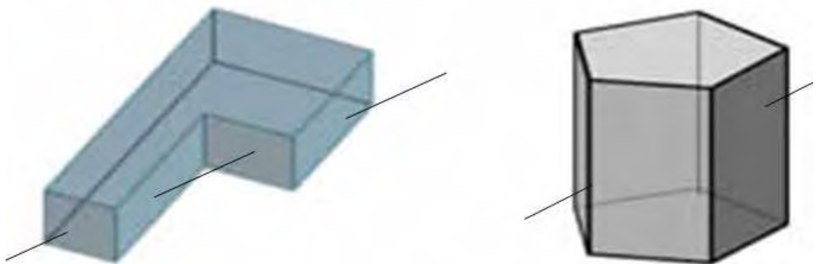
Figura 4: Poliedro não convexo e Poliedro convexo.
