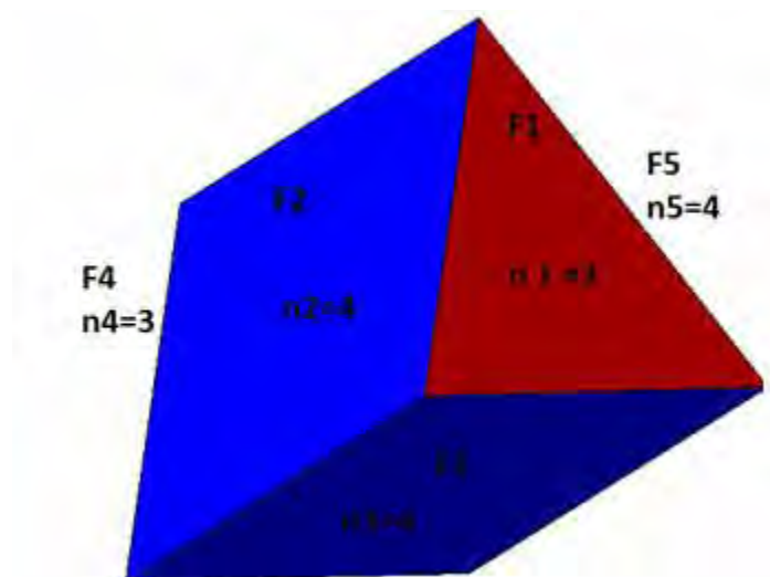
Figura 12: Prisma triangular: faces e gêneros.
