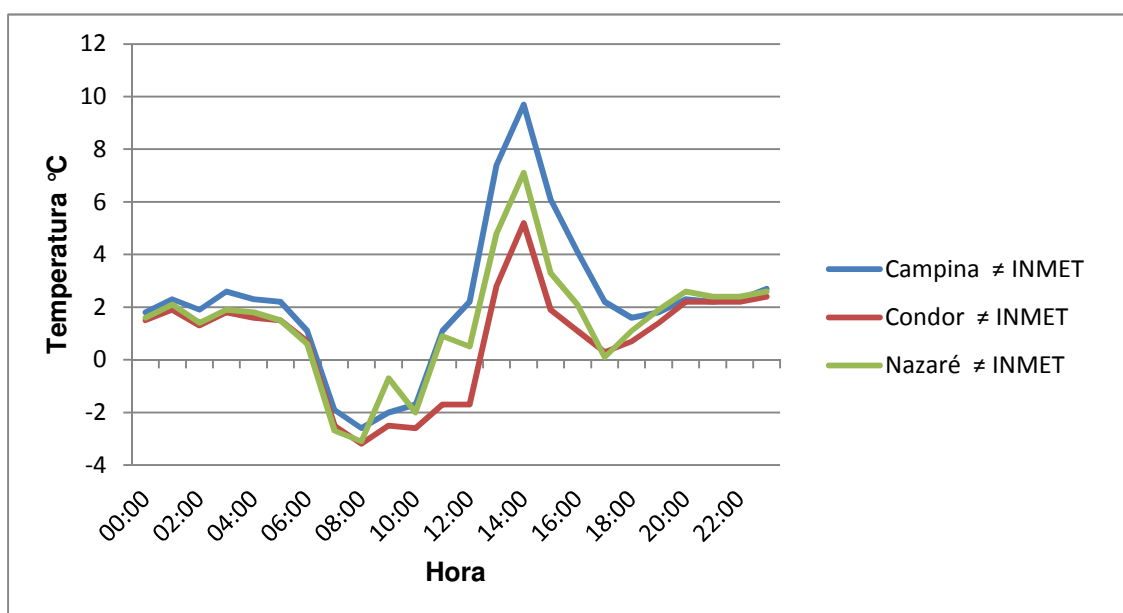
Gráfico 44 - Diferença da temperatura do dia mais quente entre os bairros da Campina, Condor e Nazaré em relação à estação do INMET (01/12/2015).
