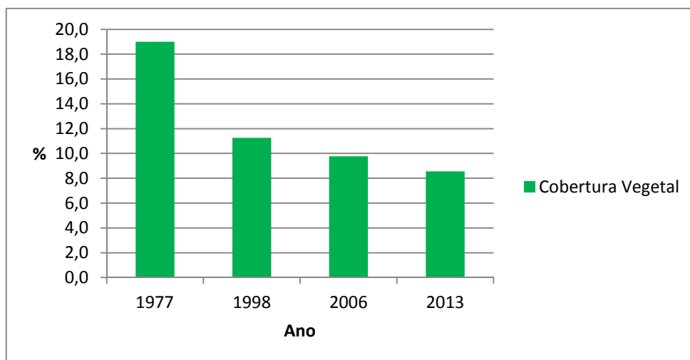
Gráfico 02 - Representação do Índice da Cobertura Vegetal em % da Primeira Légua Patrimonial de Belém-Pa (1977, 1998, 2006, 2013).
