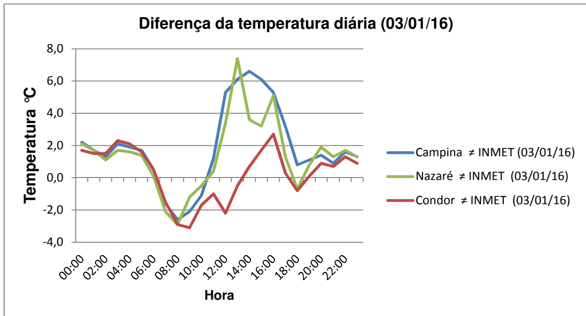
Gráfico 47 - Diferença da temperatura do dia mais quente entre os bairros da Campina, Condor e Nazaré em relação à estação do INMET (03 e 18 /01/2016).
