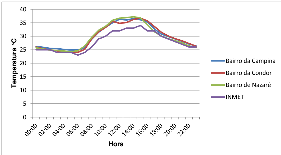
Gráfico 34 - Registro da temperatura do dia mais quente no bairro de Nazaré (30/08/15).
