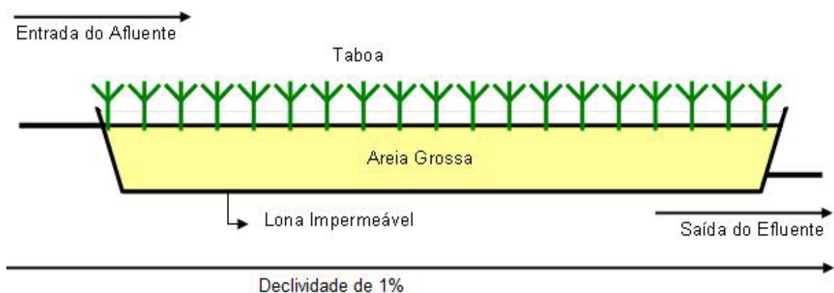
Figura 2. Desenho esquemático do segundo sistema de alagados construídos com plantas emergentes com o fluxo horizontal.
