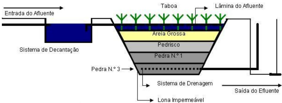
Figura 1. Desenho esquemático do primeiro sistema de alagados construídos com plantas emergentes com fluxo vertical.
