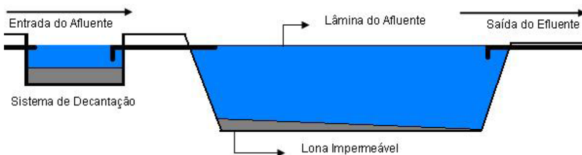
Figura 3. Desenho esquemático da lagoa facultativa.
