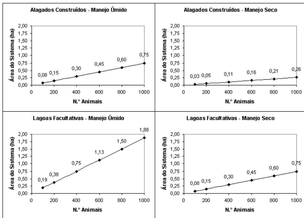
Figura 4. Área necessária para implantação dos sistemas naturais de tratamento de dejetos para suinocultura.
