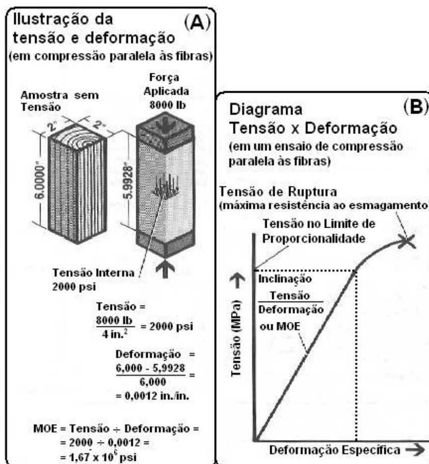
Figura 3. Ilustração de ensaio de compressão paralela às fibras (A) e diagrama de tensão deformação específica (B) (adaptado de HAYGREEN e BOWYER, 1996).
