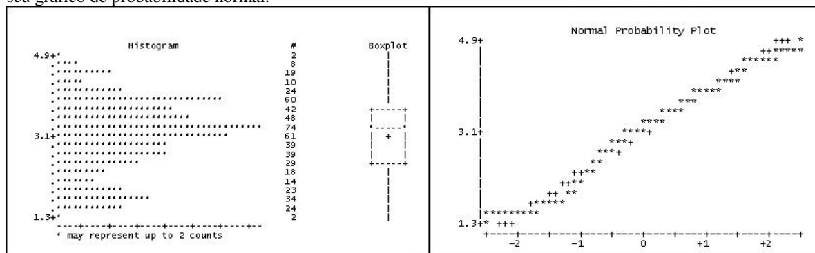
Figura 4-7: Histograma com a frequência dos dados de inchamento volumétrico na condição de 21°C-65%UR e o seu gráfico de probabilidade normal.
