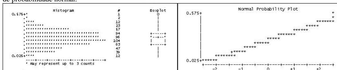
Figura 4-16: Histograma com a frequência dos dados de inchamento linear longitudinal máximo e o seu gráfico de probabilidade normal.
