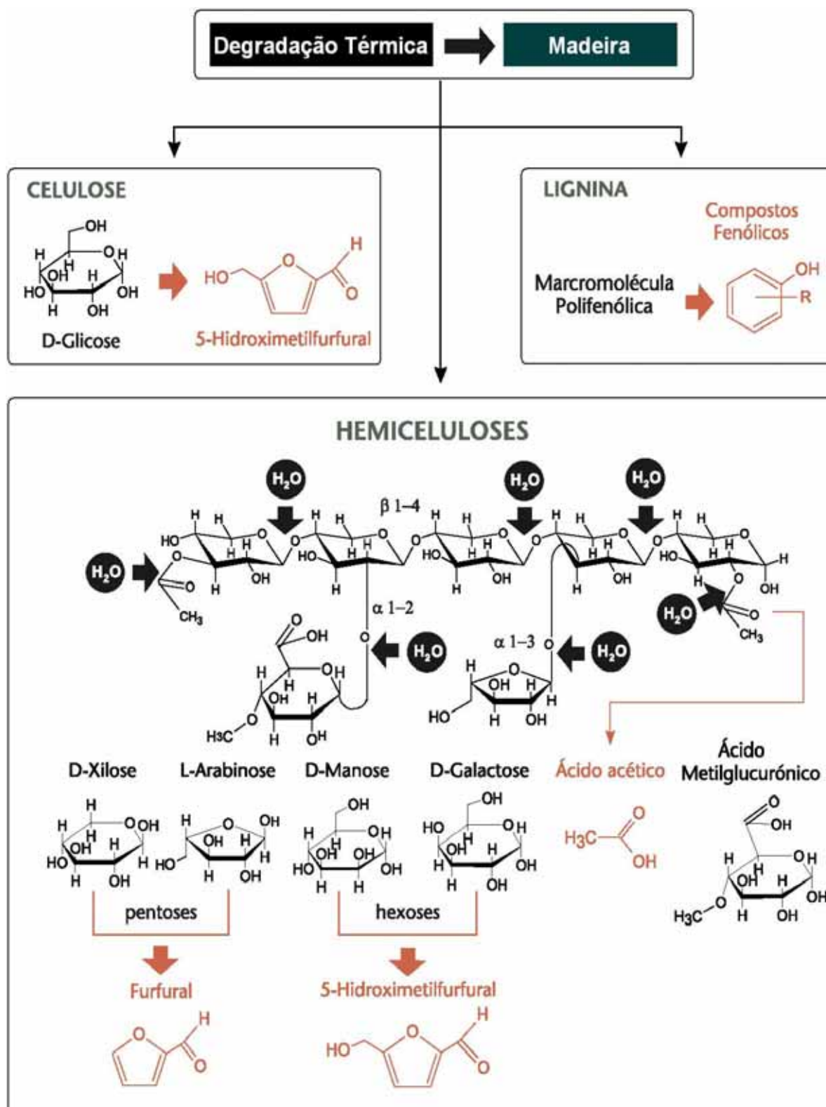
Figura 4. Degradação térmica da madeira (MARTON et al., 2003).
