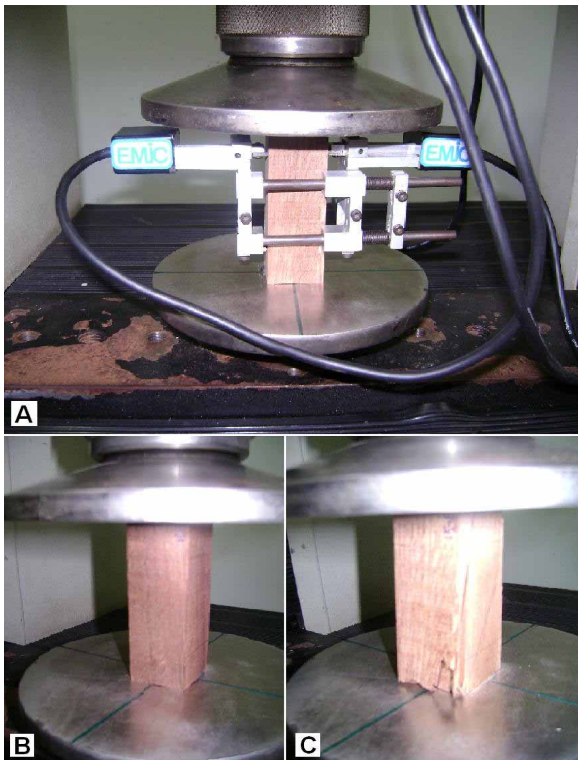
Figura 15. Execução do ensaio de compressão paralela nos corpos-de-prova: (A) detalhe do acoplamento do extensômetro; (B) retirada do extensômetro; (C) ruptura do corpo-de-prova.
