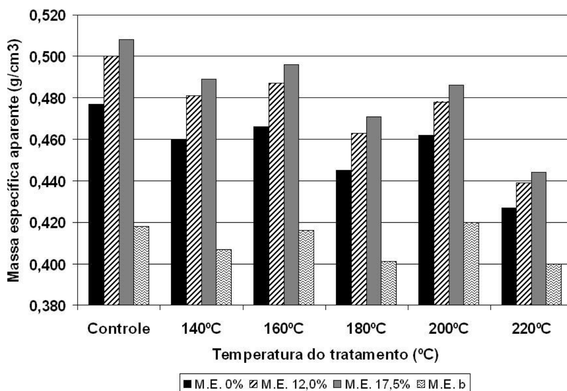
Figura 21. Efeito da termorretificação nas massas específicas aparentes da madeira de E. grandis .
