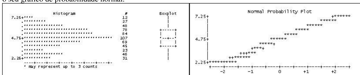
Figura 4-12: Histograma com a frequência dos dados de inchamento linear longitudinal na condição de 23°C-83%UR e o seu gráfico de probabilidade normal.
