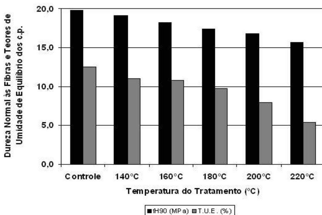
Figura 30. Efeito da termorretificação na dureza Janka normal às fibras da madeira de E. grandis .
