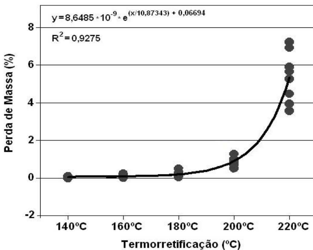
Figura 20. Regressão exponencial ajustada para estimar a perda de massa de tábuas de E. grandis em função da temperatura de termorretificação.
