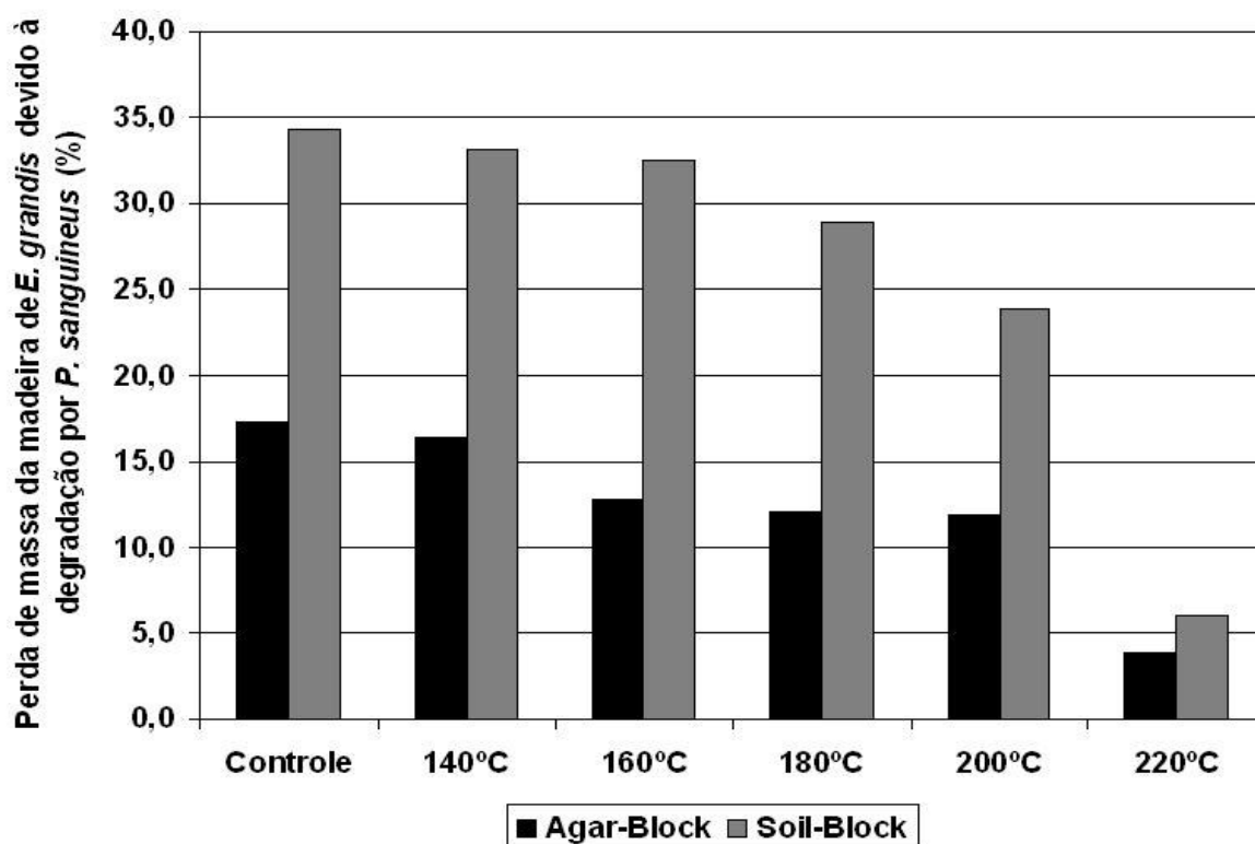
Figura 27. Perda de massa da madeira de E. grandis mediante ao fungo deteriorador P. sanguineus , em função da temperatura de termorretificação.
