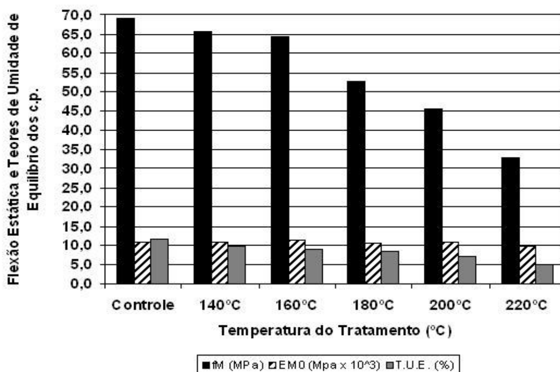
Figura 29. Efeito da termorretrificação na rigidez e resistência em flexão estática da madeira de E. grandis .
