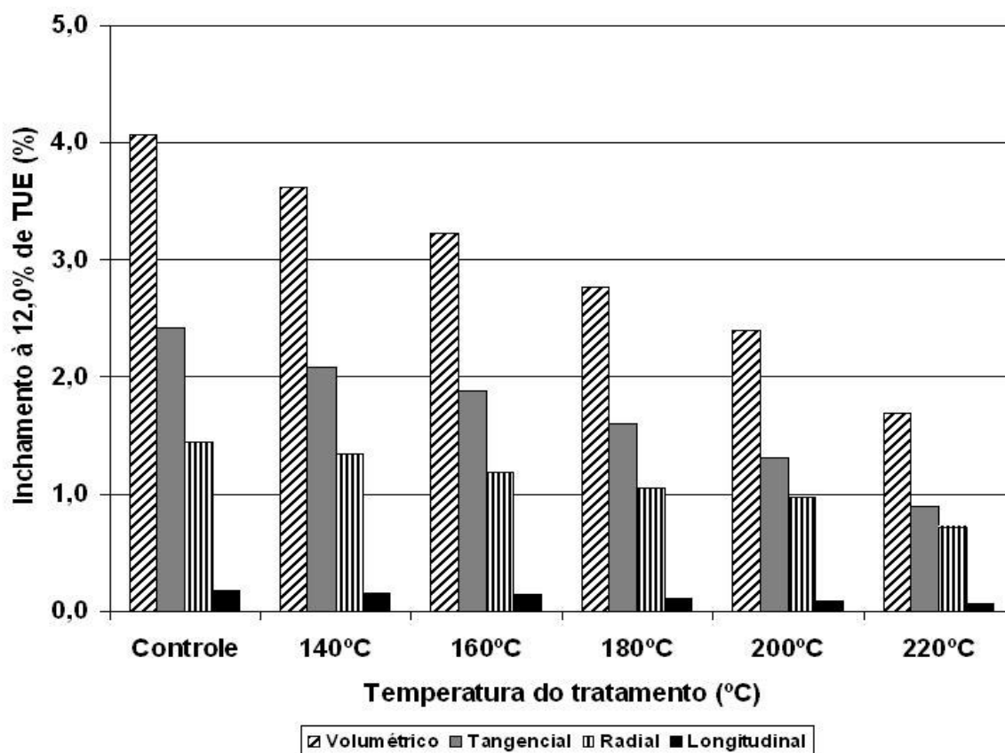
Figura 23. Efeito da termorretrificação nos inchamentos volumétricos e lineares da madeira de E. grandis climatizada a 12,0% de TUE.
