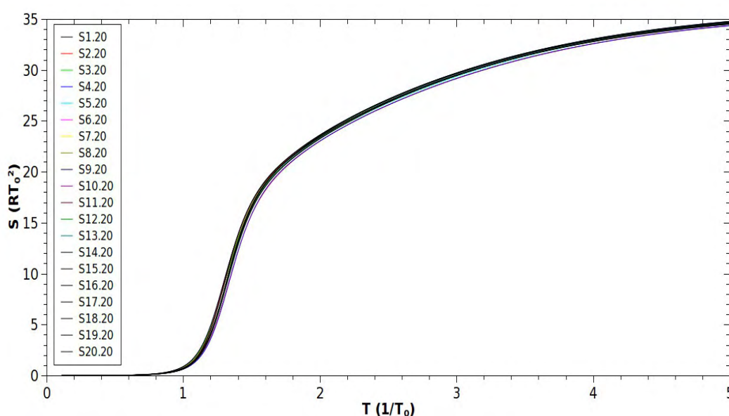
Fig. 4.7 - Entropia em função a temperatura para o conjunto de sequências do modelo de vinte letras.
