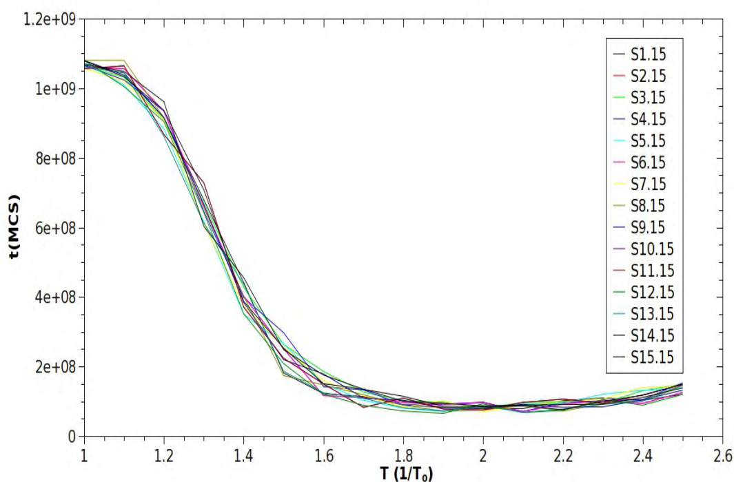
Fig 4.15 – Tempo de enovelamento das 15 cadeias com as sequências de monômeros selecionadas em função da temperatura para o modelo de 15 letras.
