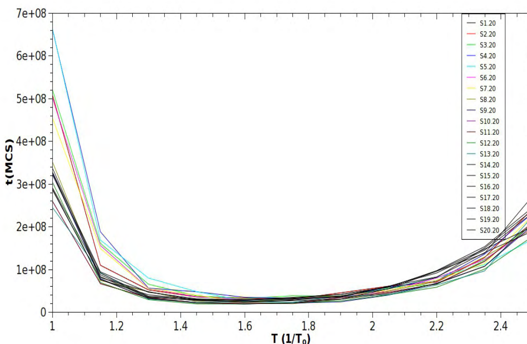
Fig 4.8 - Gráfico de tempo de enovelamento por temperatura para o conjunto de sequências compostas por 20 tipos de aminoácidos.
