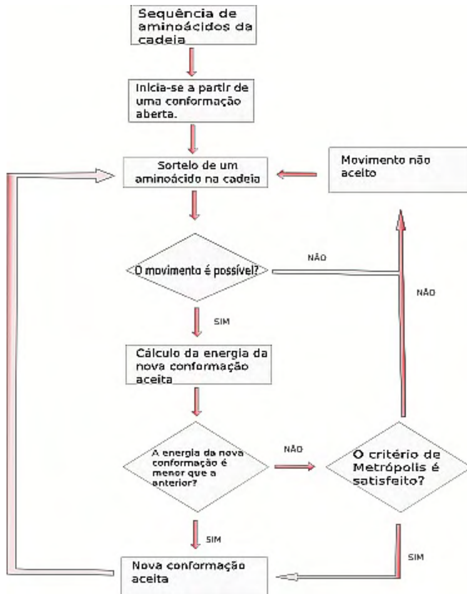
Fig. 2.10 – Fluxograma do método de metrópolis para o problema do enovelamento de proteínas.
