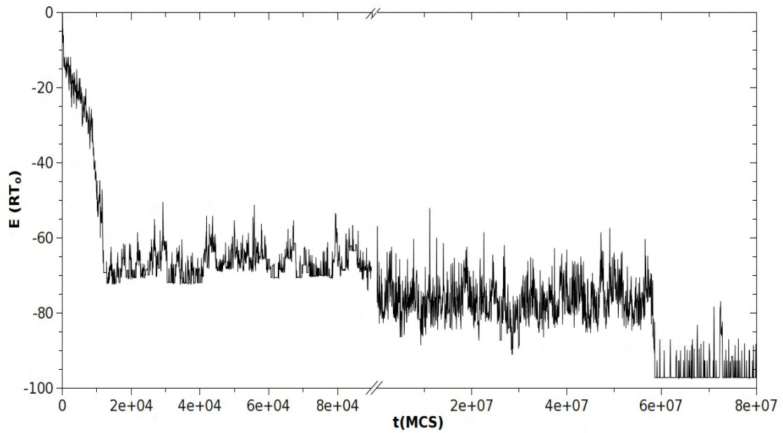
Fig 4.10 – Energia em função do tempo de enovelamento em Monte Carlo steps para a sequência S7.20 a temperatura T=1,3 .
