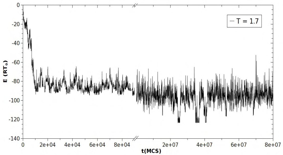
Fig 4.17 – Evolução da energia durante o enovelamento da cadeia com a sequência S2.15
