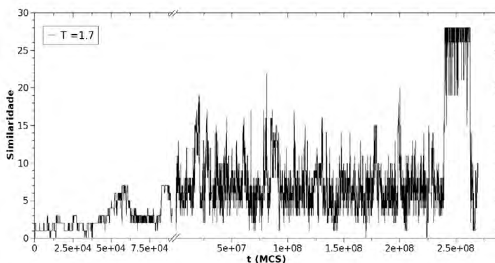
Fig 4.18 – Evolução do parâmetro de similaridade durante o enovelamento da cadeia S2.15.
