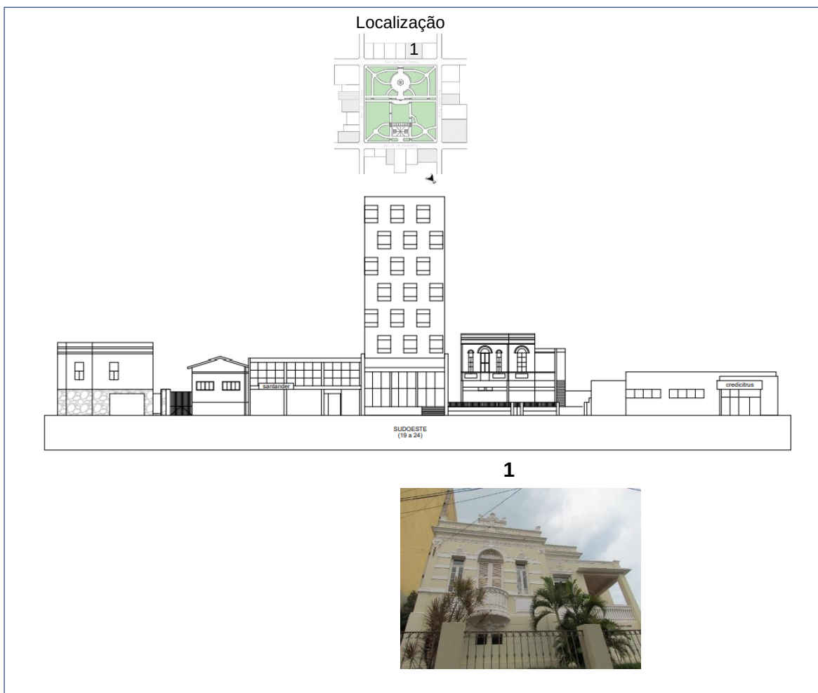
Figura 142: Estudo das fachadas e principais edificações da Rua Epitacio Pêsoa
